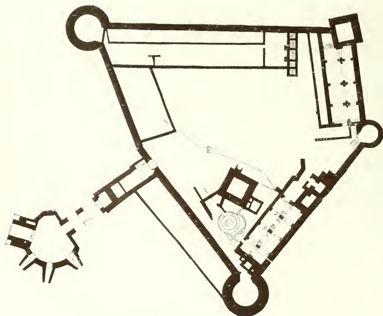
A bácsi vár alaprajza és kapuja.
