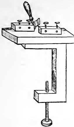
Fig. 28. Du Bois Reymond's Key.
