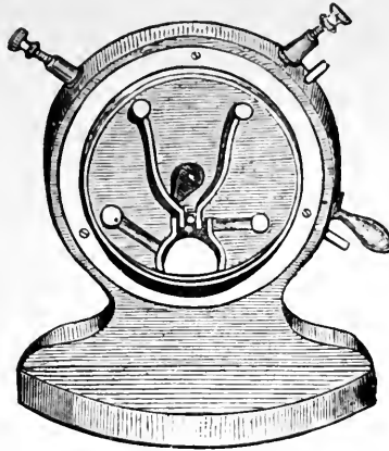
Fig. 33. Commutator.
