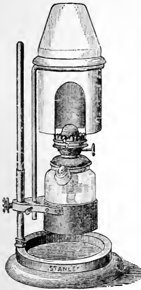
Fig. 6.—Microscope Lamp.
