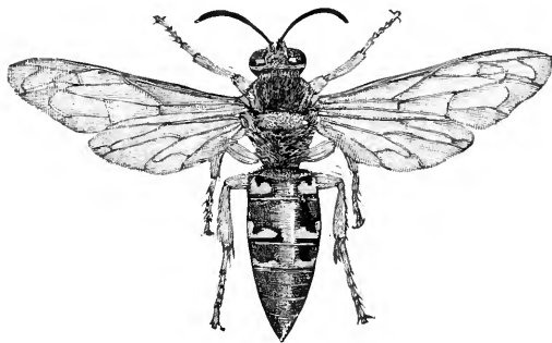
FIG. 778.— Sphecius speciosus .
