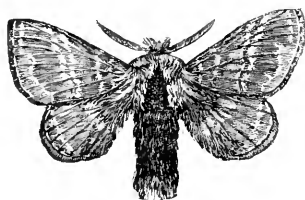
FIG. 443.— Tolyte velleda .
