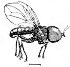
FIG. 577.— Pipunculus .
