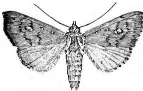
FIG. 361.— Aletia argillacea .
