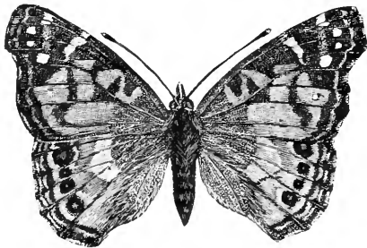
FIG. 474.— Vanessa huntera .
