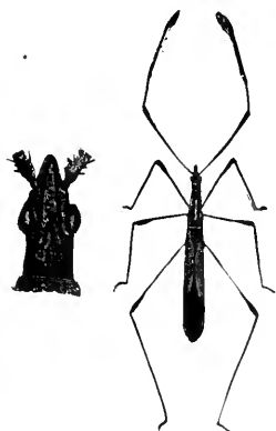
FIG. 175.— Jalysus spinosus .
