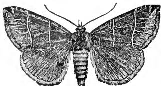
FIG. 355.— Parallelia bistriaris .
