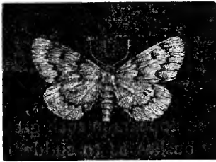
FIG. 331.— Cleora semiclusaria .
