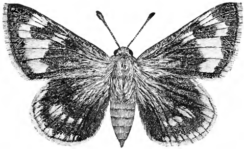
FIG. 448.— Megathymus cofaqui .
