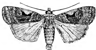
FIG. 371.— Noctua c-nigrum .
