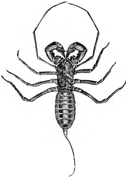
FIG. 11.— Thelyphonus giganteus .
