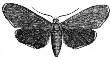
FIG. 401.— Ctenucha virginica .
