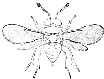
FIG. 760.— Aphycus eruptor .
