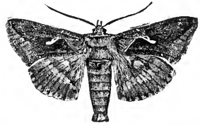
FIG. 360.— Plusia simplex .
