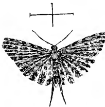
FIG. 285.— Orneodes hexadactyla .
