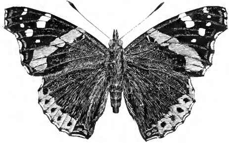
FIG. 473.— Vanessa atalanta .
