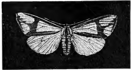
FIG. 388.— Haploa contigua .
