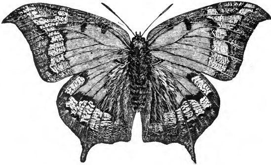
FIG. 480.— Anæa andria .
