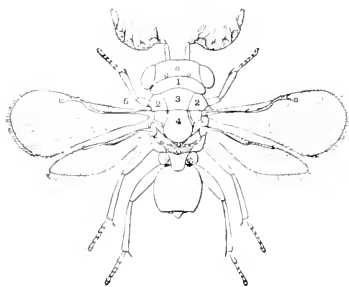
FIG. 759.— Dilophogaster californica .
