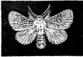
FIG. 246.— Megalopyge crispata .
