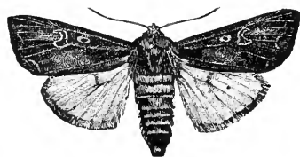
FIG. 370.— Mamestra picta .
