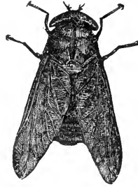
FIG. 540.— Tabanus atratus .
