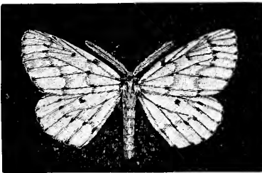
FIG. 330.— Cingilia catenaria .
