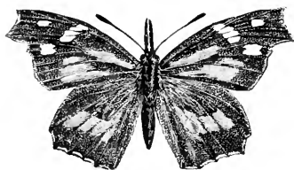
FIG. 468.— Hypatus bachmanni .
