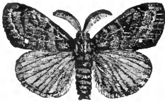
FIG. 376.— Notolophus leucostigma .
