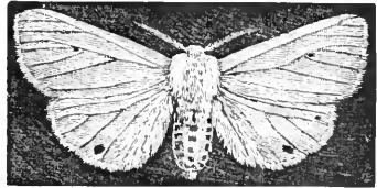
FIG. 395.— Spilosoma virginica .
