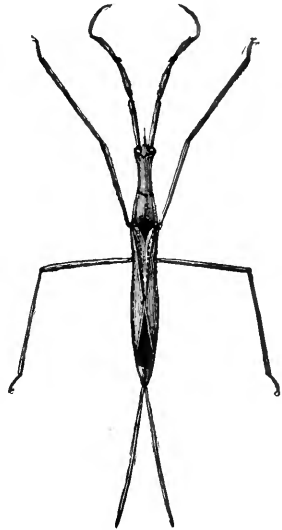
FIG. 150.— Ranatra fusca .
