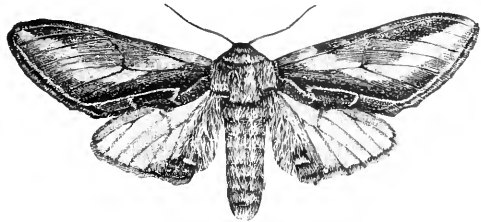
FIG. 310.— Pheosia rimosa .
