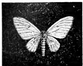
FIG. 340.— Dyspteris abortivaria .
