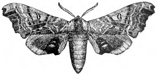
FIG. 410.— Smerinthus geminatus .
