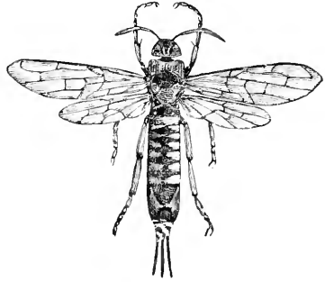
FIG. 744.— Tremex columba .
