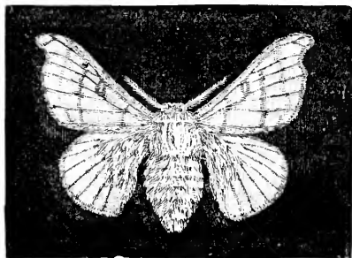
FIG. 418.— Bombyx mori .
