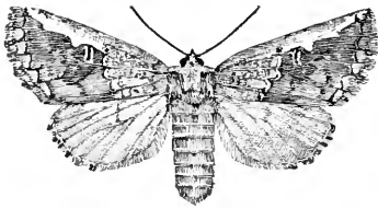
FIG. 314.— Edema albifrons .
