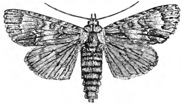
FIG. 372.— Acronycta morula .
