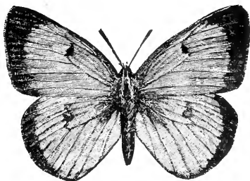
FIG. 464.— Eurymus philodice .
