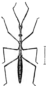
FIG. 158.— Linnobates lineata .
