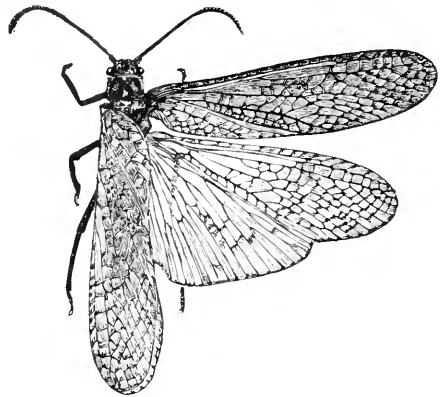
FIG. 103.— Pteronarcys regalis .
