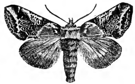
FIG. 348.— Thyatira scripta .
