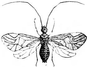
FIG. 107. — PSOCUS VENOSUS.
