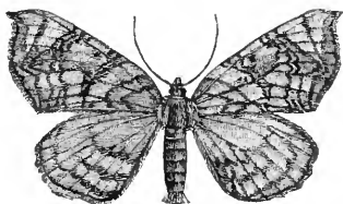
FIG. 338.— Eustroma diversilineata .
