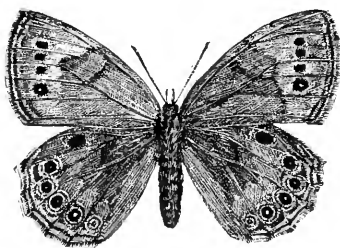
FIG. 481.— Satyroides eurydice .
