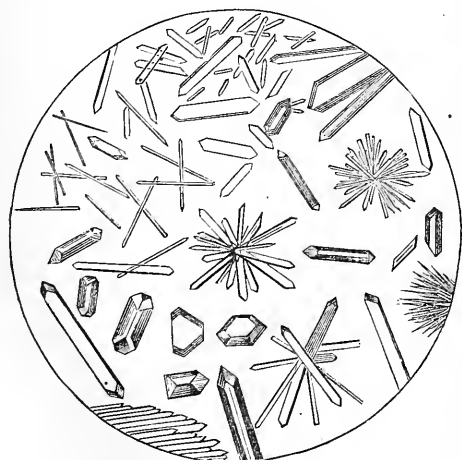
Fig. 195. Hippuric Acid.
