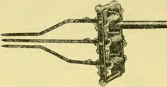
FIG. 27. TRIPLE TIME-MARKER.
