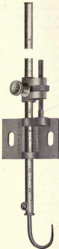
FIG. 111 No. 628 HOOK GAGE
