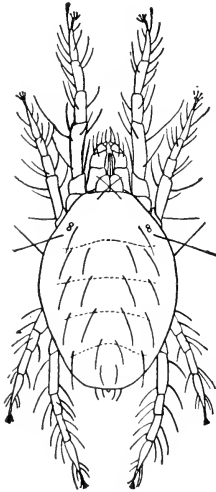
FIG. 221. — The red-spider ( \times 66 ).
