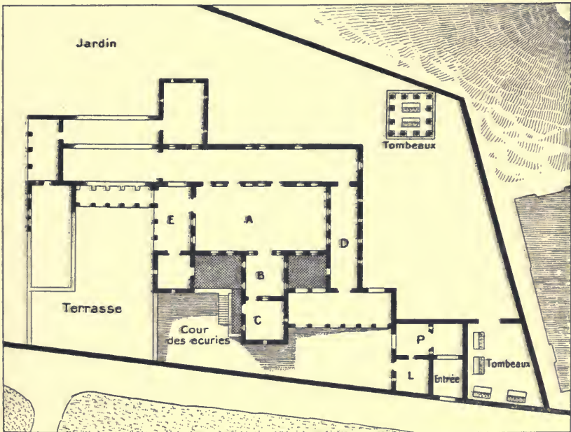
107. — Villa d'El Barah, d'après de Vogüé, Syrie centrale , pl. 51.
