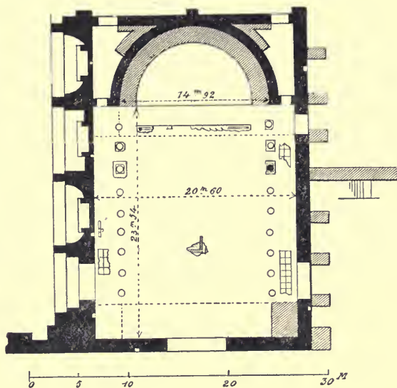
114. — Plan de la basilique privée de la domus Flaviorum , d'après Lange, Haus und Halle , pl. vi, fig. 2.
