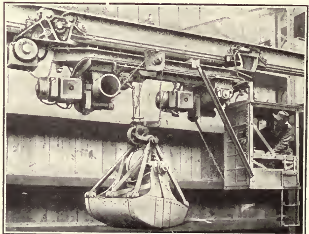
Grab-Bucket Hoist
