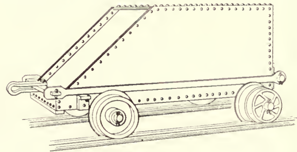
Fig. 64—Skip Car
