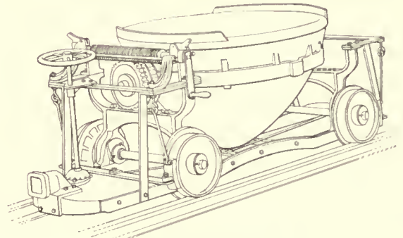
Fig. 71—Smelter Slag Car
