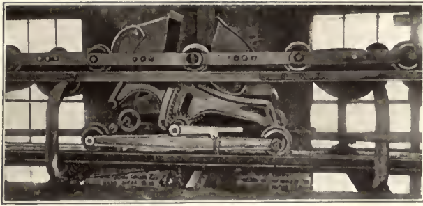
Discharger
