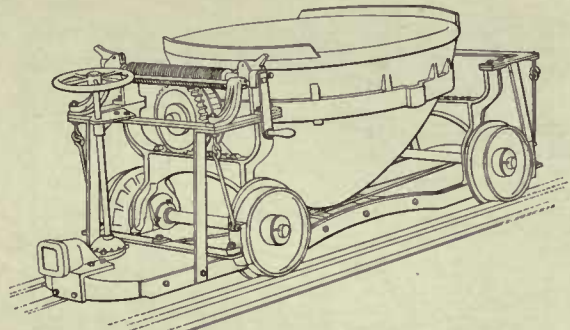
Fig. 74—Smelter Slag Car
