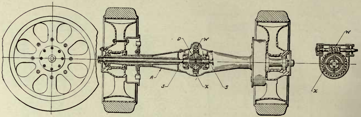
Fig. 12—Worm Drive
