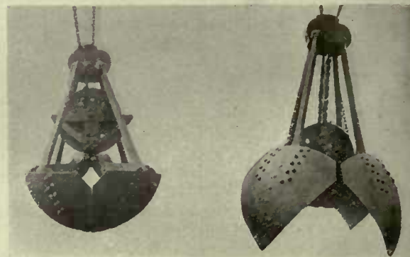
ORANGE PEEL BUCKET—4 BLADES
