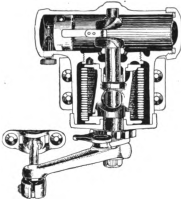
FIG. 128. Check valve.
