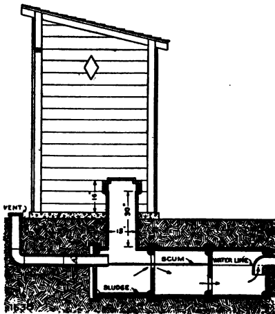
FIG. 81-a. Septic tank.
