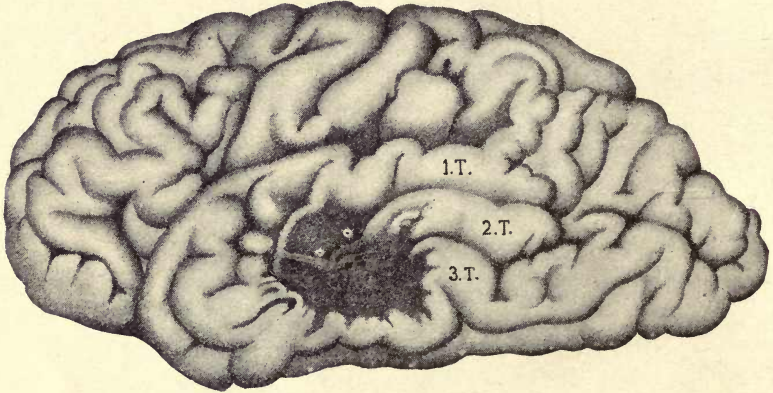
Fig. 21—Left hemisphere
