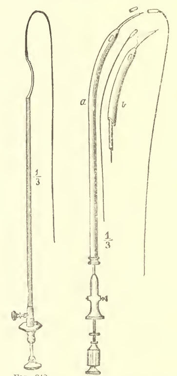
FIG. 342.—Urethrotome of M. MALLEZ. FIG. 343.—CHARRIÈRE'S urethrotome porte-sonde.
