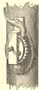
FIG. 570.—Extension pulley. [After VEDDER.]
