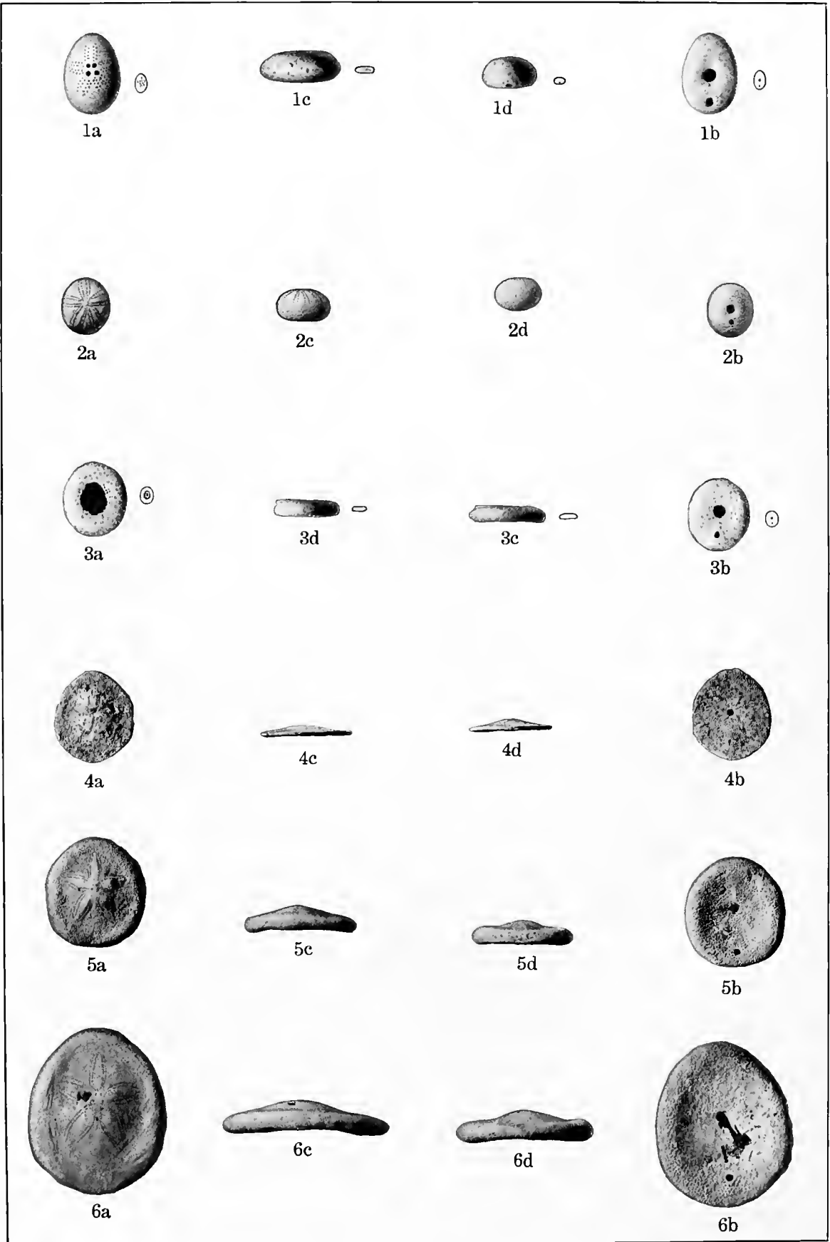
EOCENE ECHINOIDEA.
