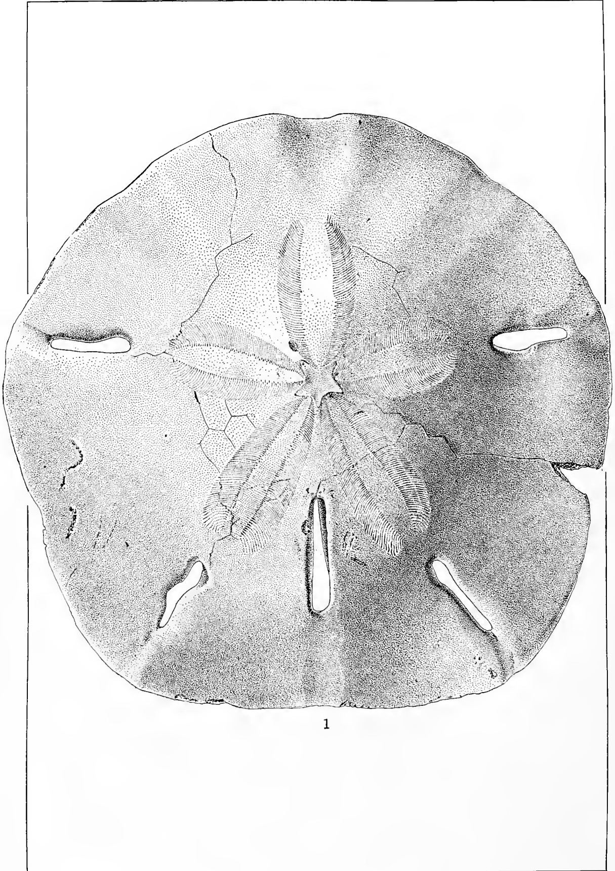
PLEISTOCENE ECHINOIDEA.
