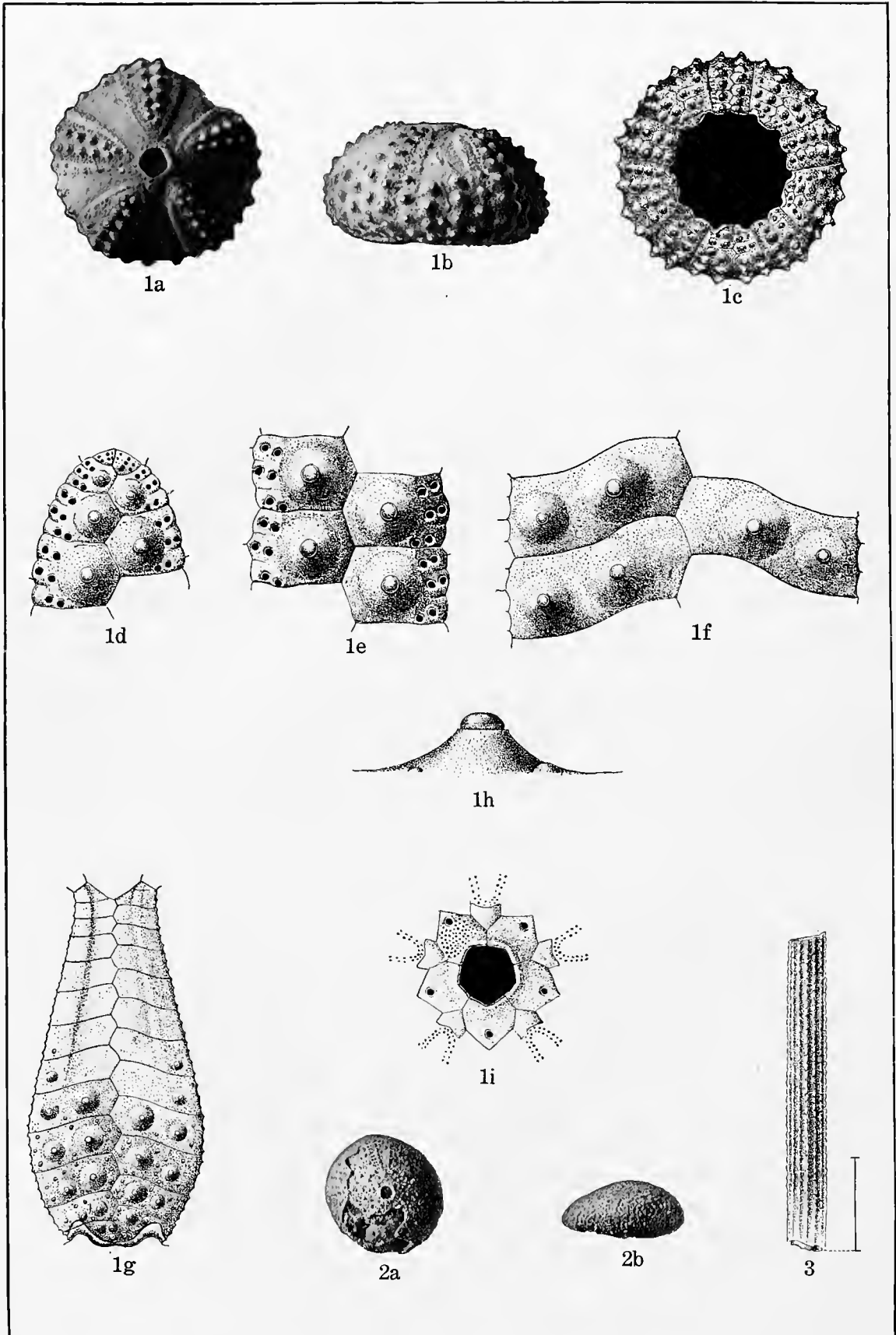
EOCENE ECHINOIDEA.
