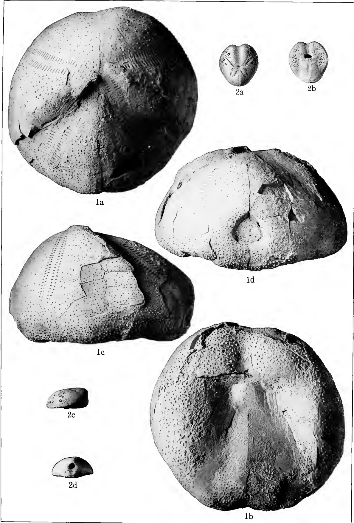
EOCENE ECHINOIDEA.
