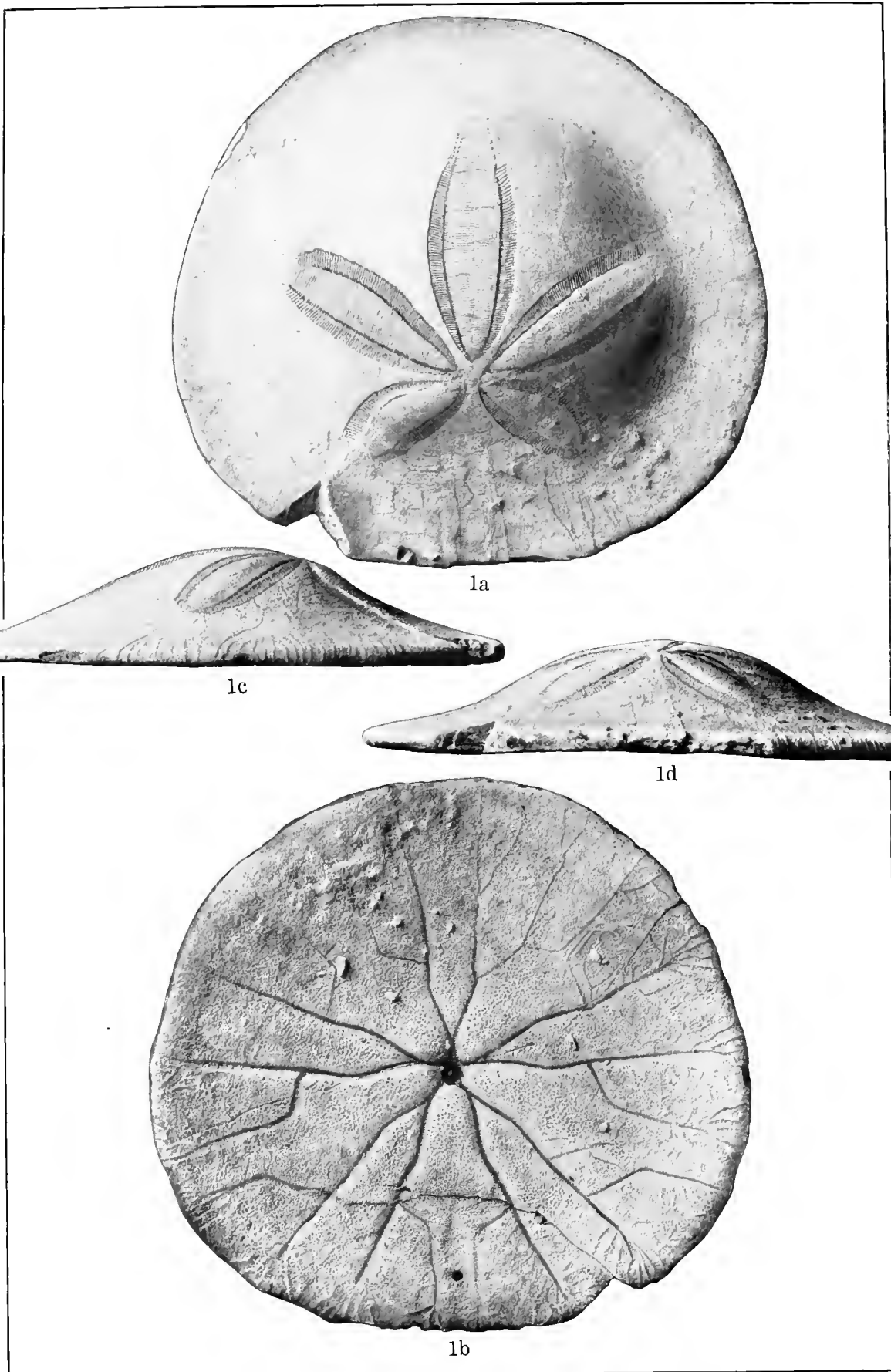
PLEISTOCENE ECHINOIDEA.
