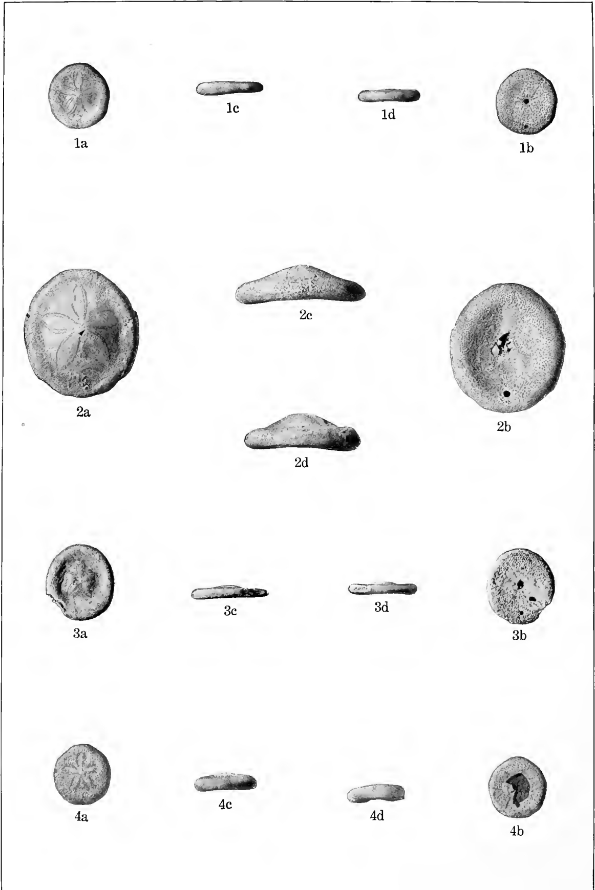
OLIGOCENE ECHINOIDEA.
