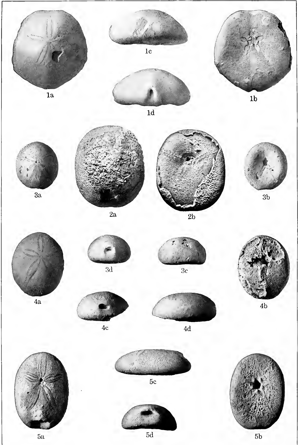
EOCENE ECHINOIDEA.
