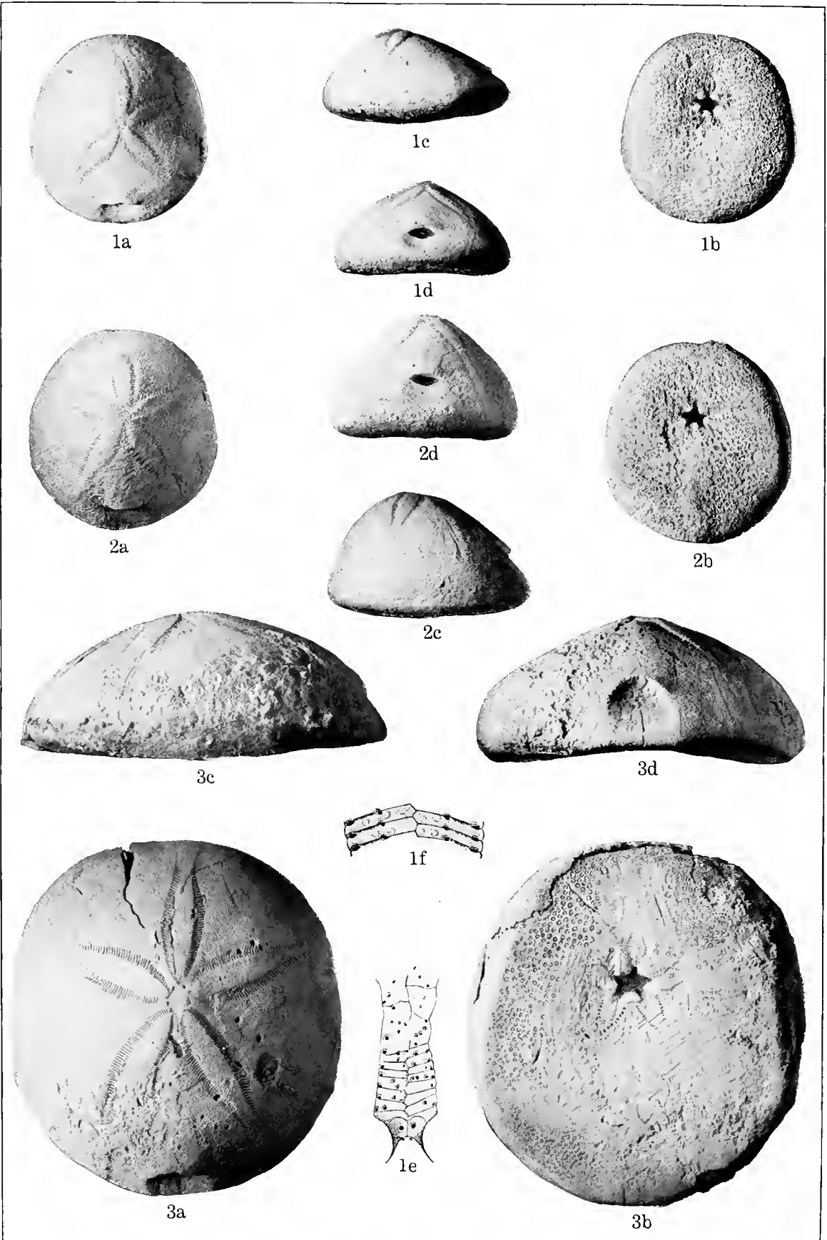
OLIGOCENE ECHINOIDEA.
