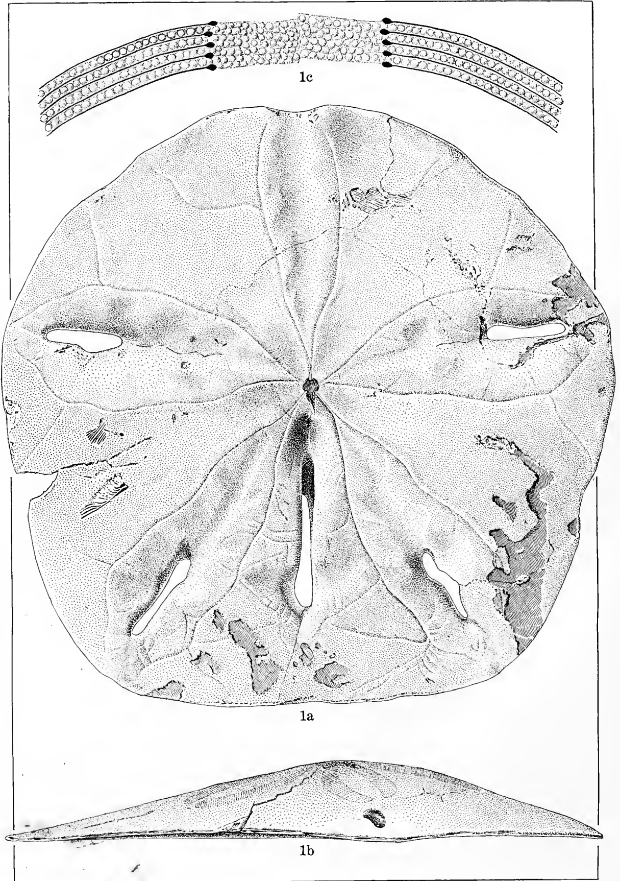
PLEISTOCENE ECHINOIDEA.
