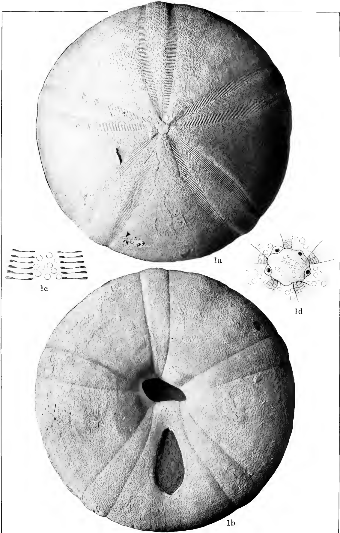
OLIGOCENE ECHINOIDEA.
