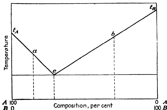
Fig. 5.—Simple eutectic diagram.
