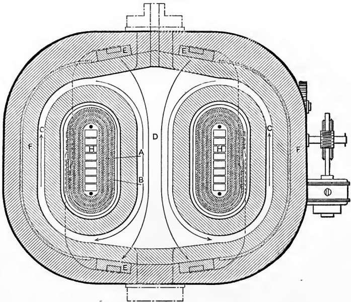
FIG. 190.—Röchling-Rodenhauser Furnace.
