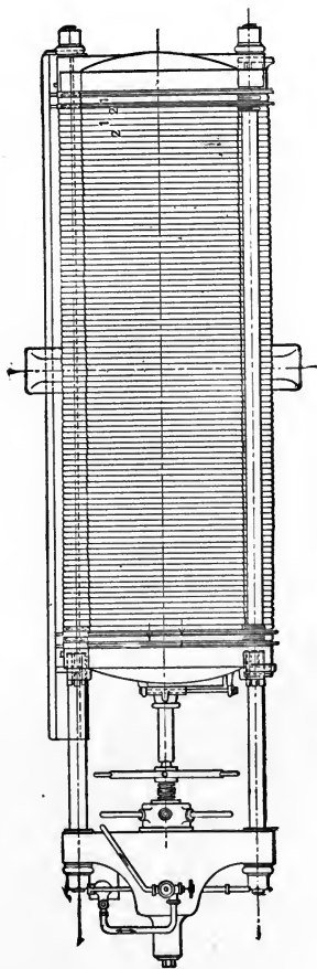
FIG. 25.—Plan. Filter Press with Iron Frames (Klein, Schanzlin & Becker, Frankenthal).
