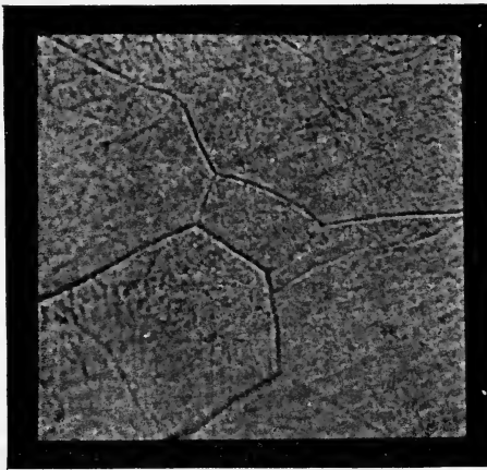
FIG. 177.—Ferrite ( \times 500 ).
