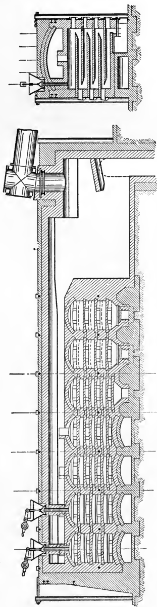
FIG. 88.—Maletra-Schaffner Furnace (Lunge). Scale, 1 : 150.
