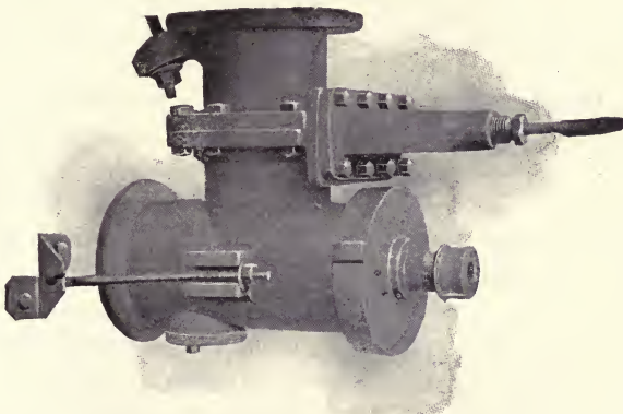
Fig. 136. TUYERE.
