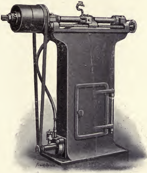
Fig. 77. ZINC LATHE.
