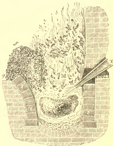
FIG. 29.—Catalan Forge.
