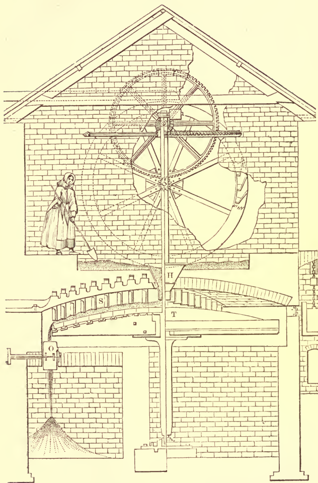
FIG. 48.—Brunton's Calciner.
