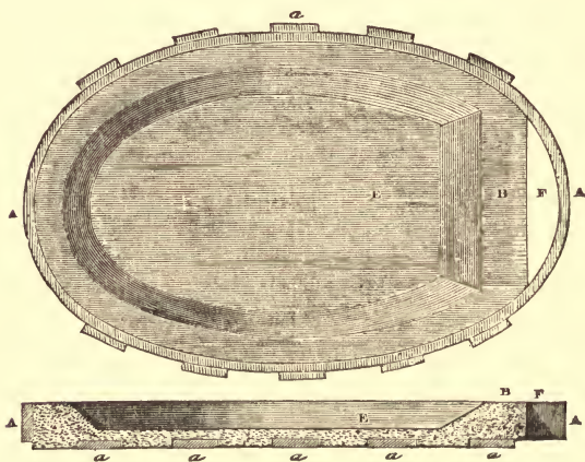
FIG. 74.—English Cupel or Test.
