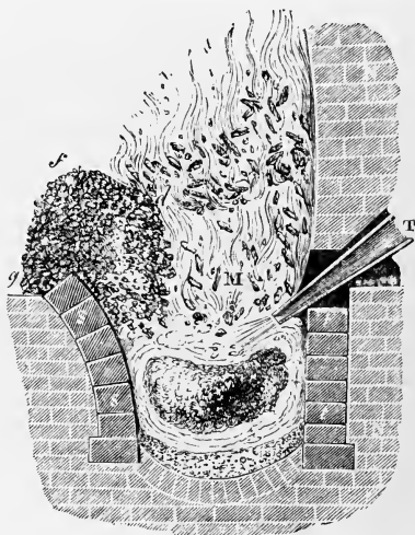
FIG. 29.—Catalan Forge.
