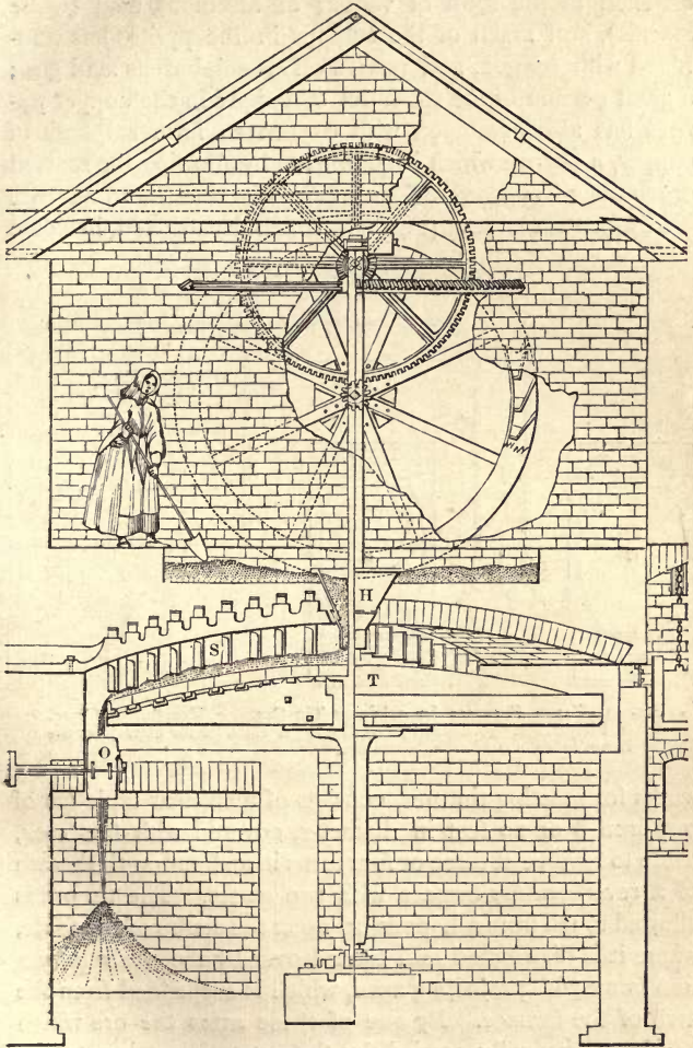
FIG. 48.—Brunton's Calciner.
