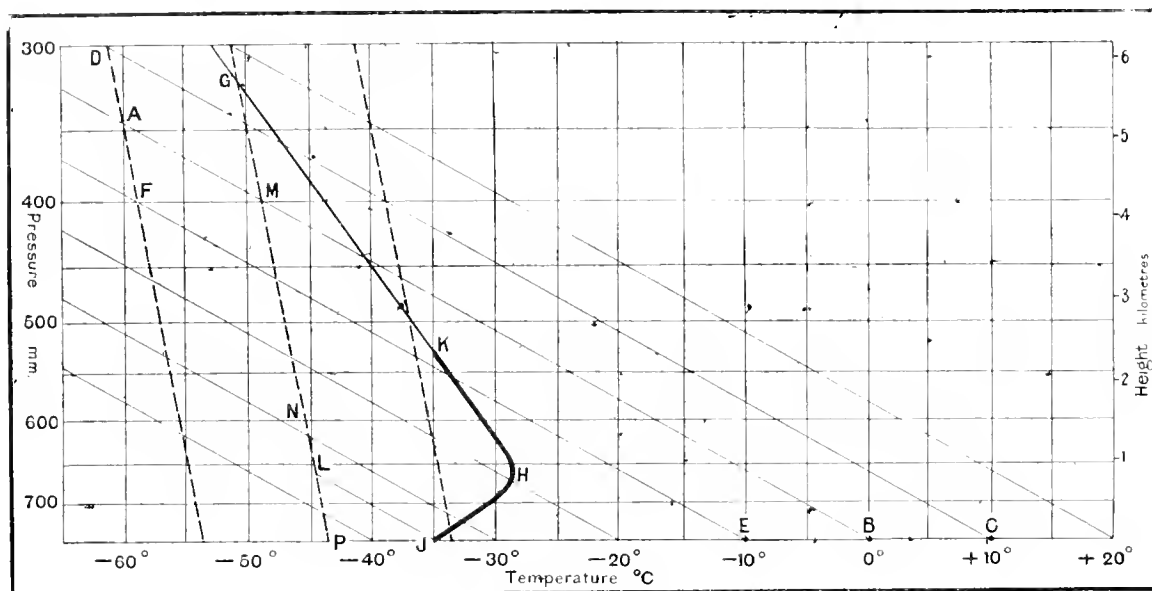
FIG. 83. Hertz diagram.
