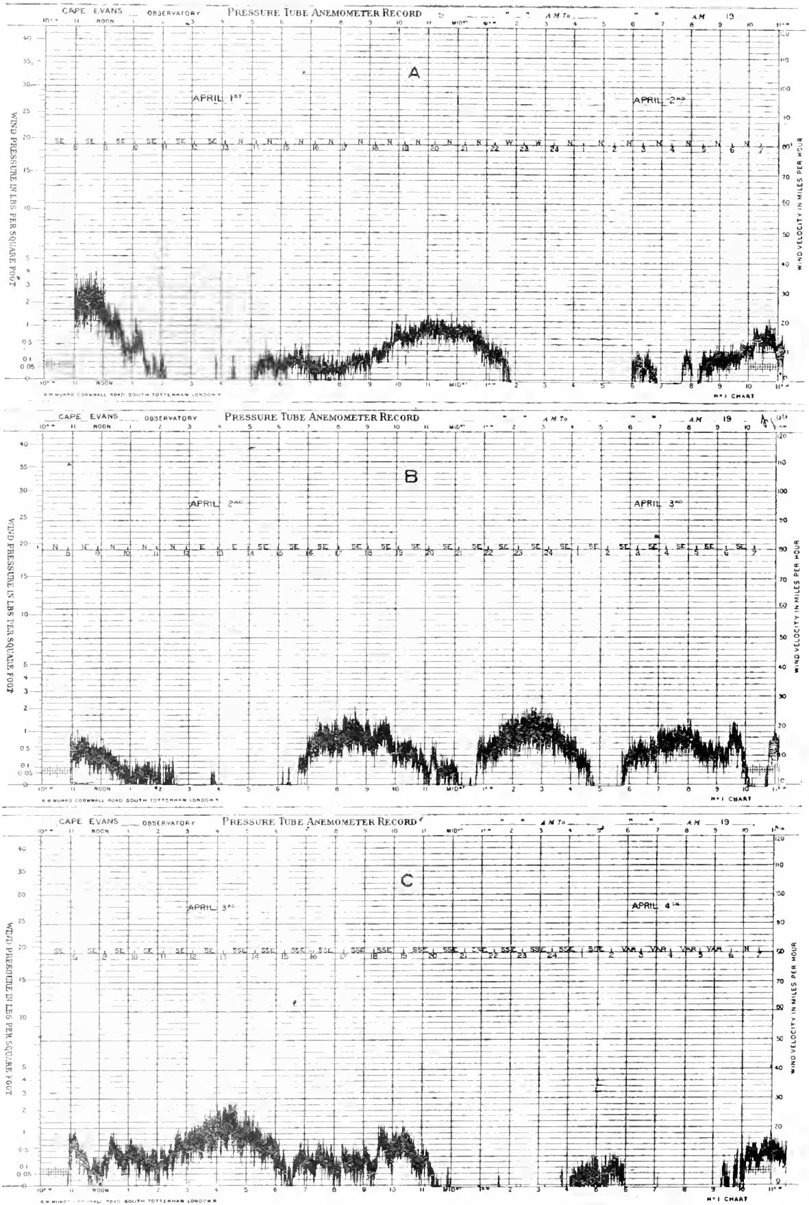
FIG. 11. Anemograms.
