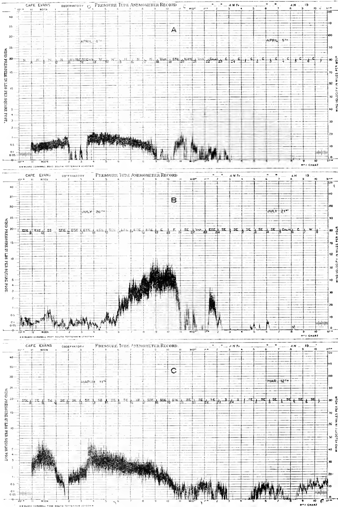
Fig. 45. Anemograms.
