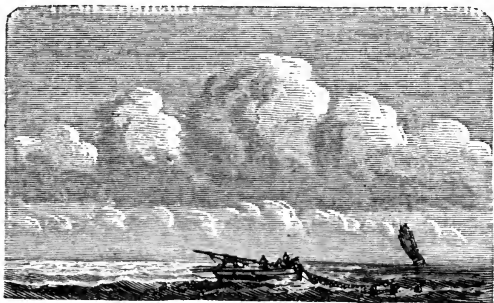
CUMULUS.
