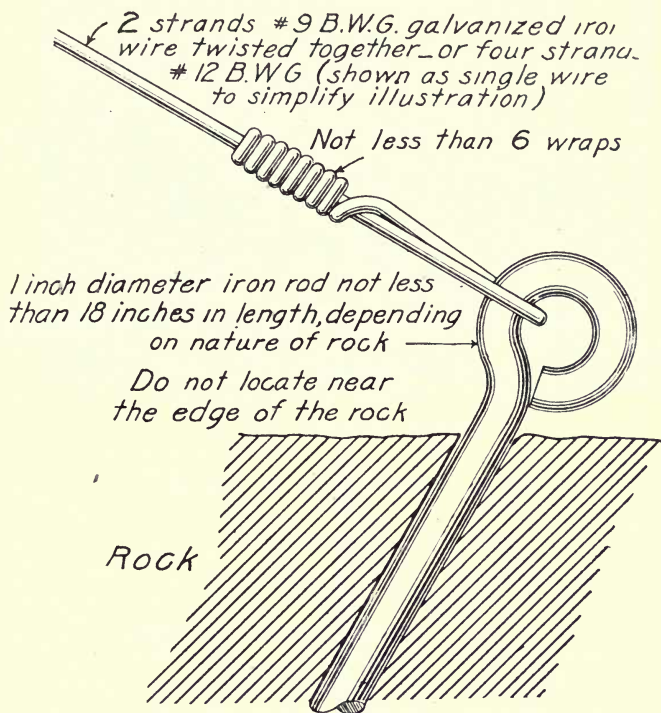
Fig. 16 Rock guy bolt
