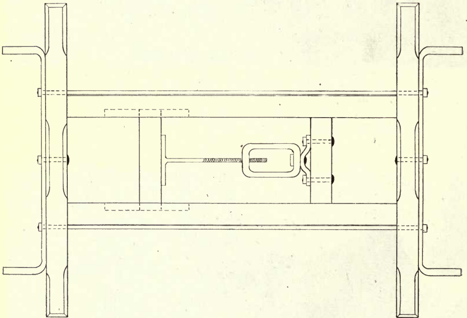
Fig. 7 Mobley wire-cradle.
