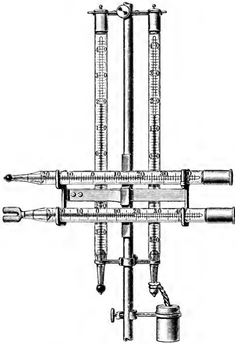
Fig. 4. Thermometer und Psychrometer.
