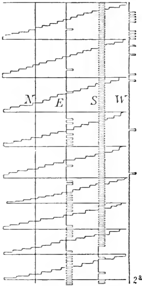
Fig. 9. Registrierprobe des Sprungigen Anemographen.
