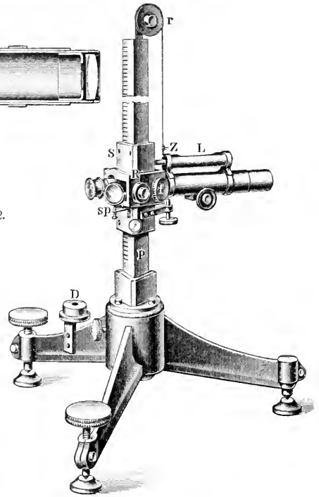
2. Kathetometer von Fueß.
