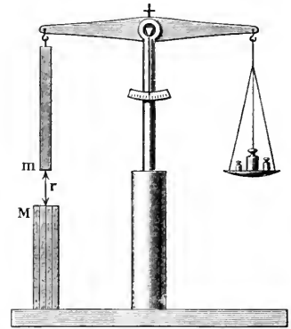
Fig. 1. Magnetische Waage.
