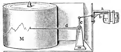
Fig. 2. Schema des Richardschen Thermographen nach Hfmann.
