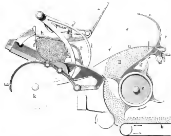
5. Bindemäher von Advance, Platt u. Comp. Querschnitt. (Vgl. Fig. 1.)
