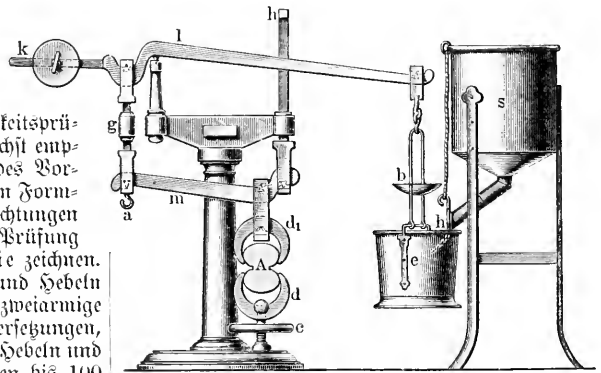
Fig. 1. Frühling's Hebelzerreißapparat.
