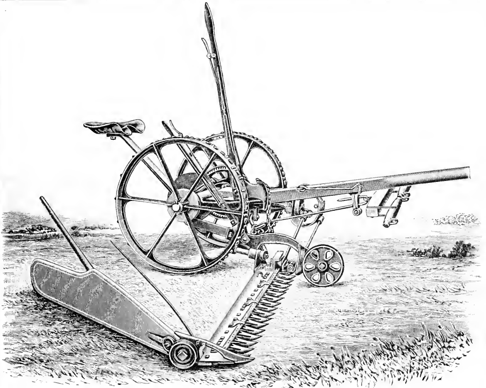
1. Grasmähmaschine von F. Zimmermann u. Komp. Halle a. S.
