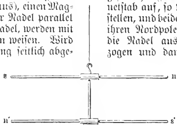
Fig. 3. Astatisches Nadelpaar.
