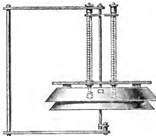
Fig. 1. Jalousievorrichtung von Köppen.
