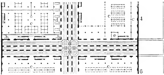
II. Östlicher Teil der Pariser Markthallen. Untergeschoß unter den Abteilungen 3—6.
