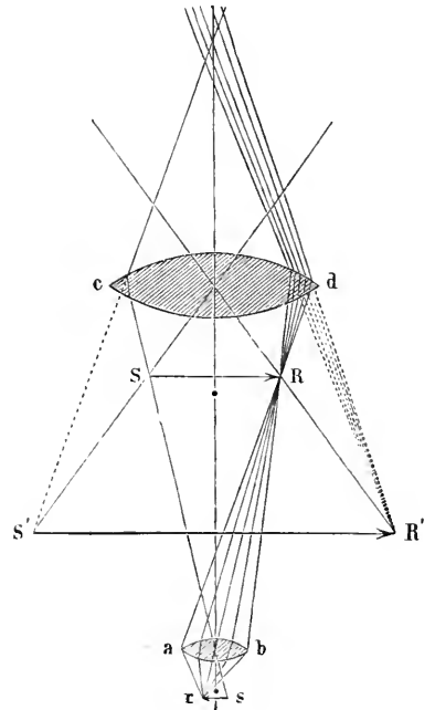
Fig. 1. Einrichtung des zusammengesetzten Mikroskops.
