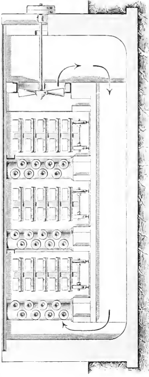
4. Kanaltrockenanlage von Möller u. Pfeifer.
