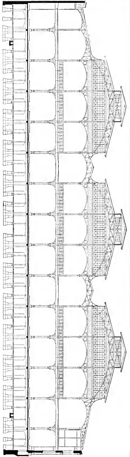
III. Zentralmarkthalle in Berlin. Durchschnitt.
