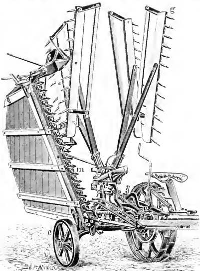
4. Getreidemähmaschine in Transportstellung der Plano Harvester Comp., Chicago.
