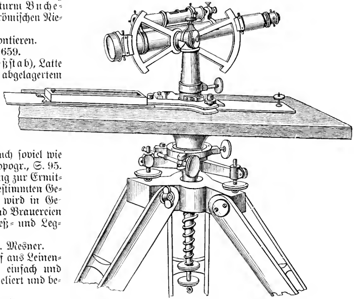
Breithaupts Normalnivelearrnat mit Kippregel.
