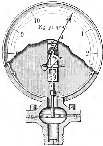
Fig. 2. Plattenfedermanometer.
