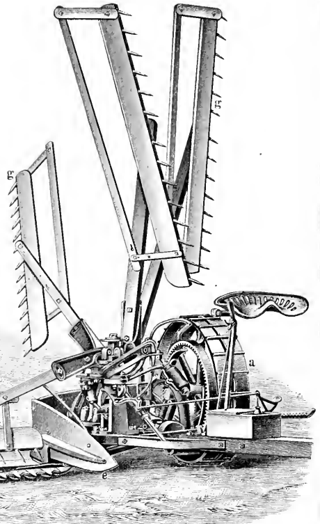
5. Getreidemähmaschine von Walter A. Wood, Hoosick Falls.
