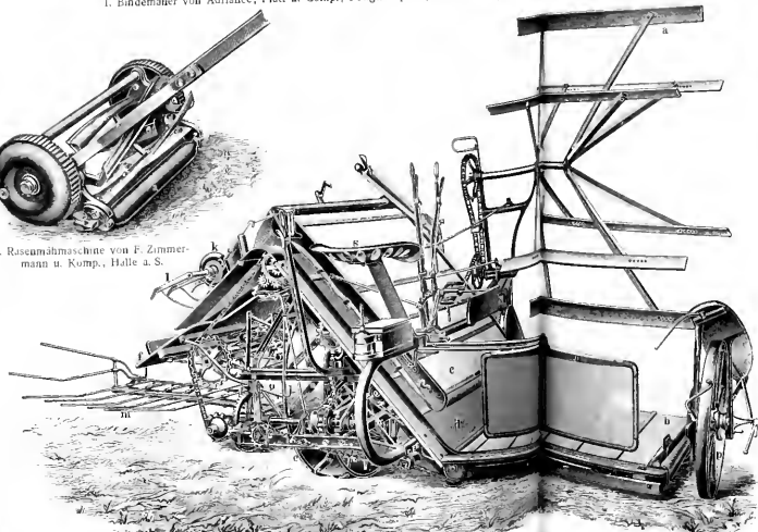
4. Bindemäher von McCormick Harvester Comp., Chicago. Bilder aus dem Katalog der Maschinenfabrik in Leipzig.
