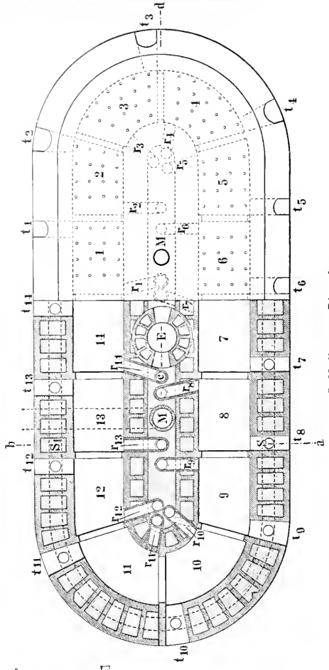
5. Hoffmann's Ringofen.
