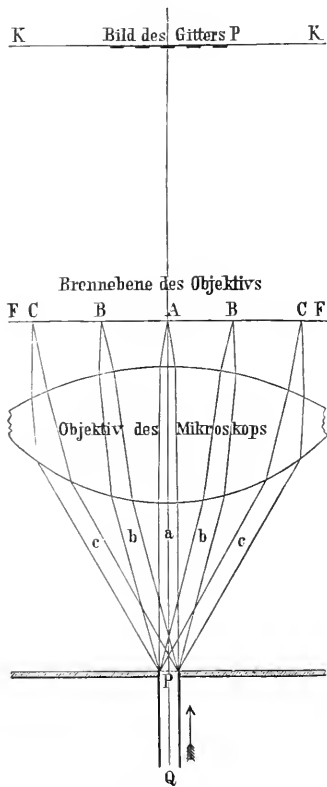
Fig. 3. Mikroskopische Bilderzeugung auf Grund der Beugungstheorie (Abbe).
