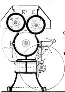
6. Schlickeysens liegende Ziegelpresse. Quer- und Längsschnitt.
