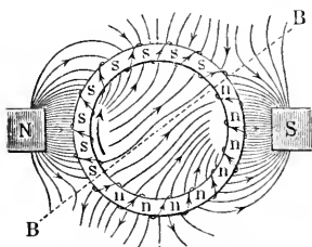
Fig. 5. Magnetfeld des bewegten Ringanters einer Dynamomaschine.
