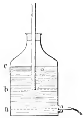
Mariottesche Flasche.
