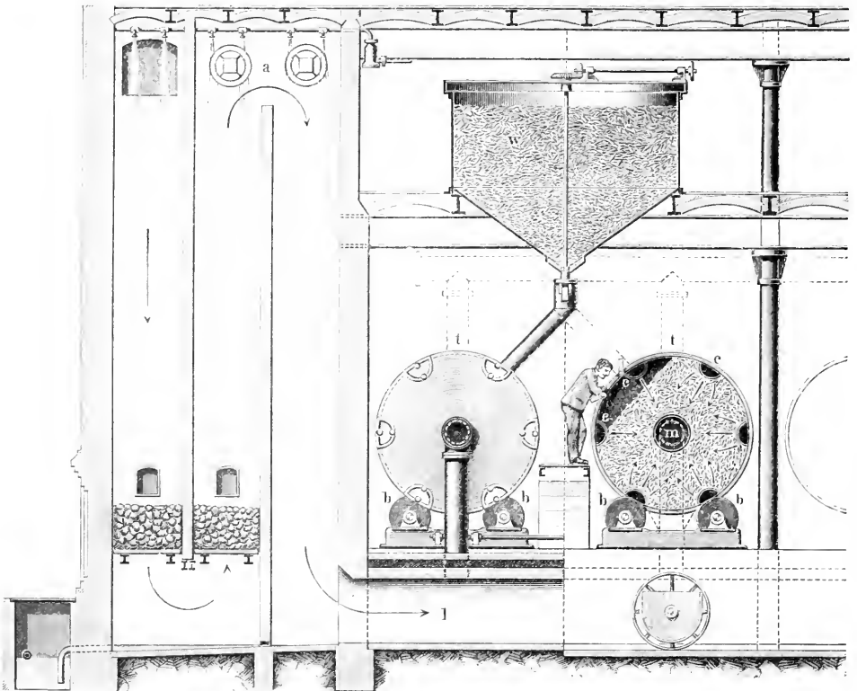
1. Gallands pneumatischer Keimapparat.
