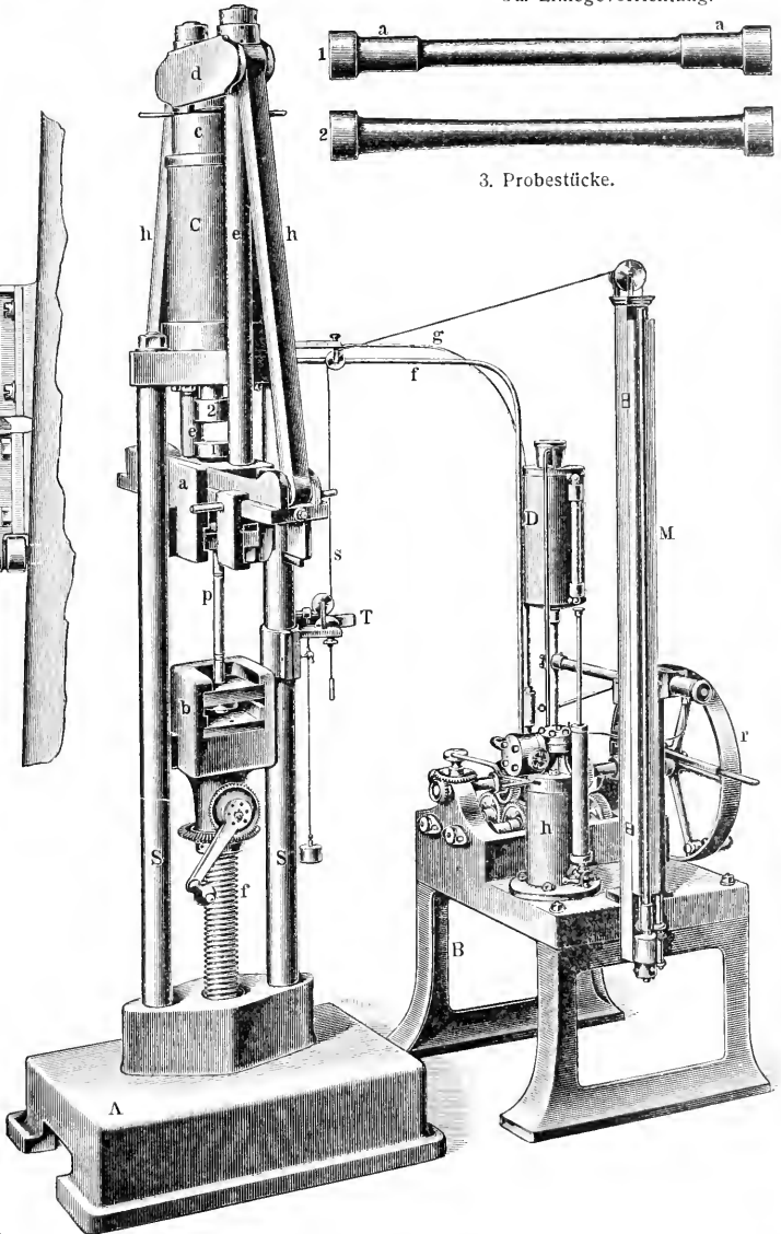
2. Zerreißmaschine mit Flüssigkeitsdruck.
