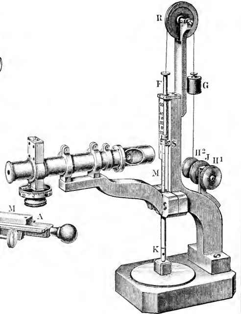
5. Kontaktmikrometer von Zeiß.
