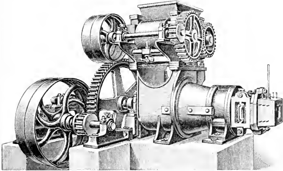
4. Ziegelmaschine von Röhrig u. König.
