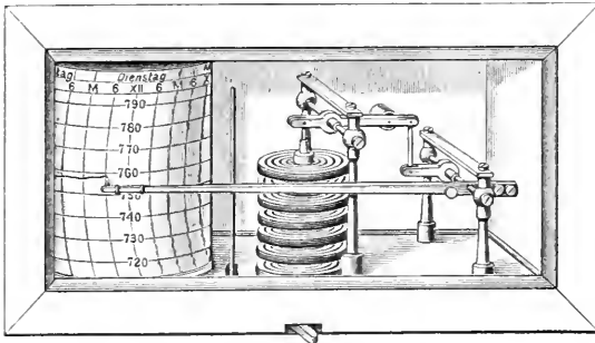
Fig. 3. Richardscher Barograph.
