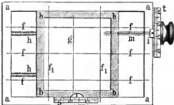
Fig. 2. Faden- oder Schraubemikrometer.
