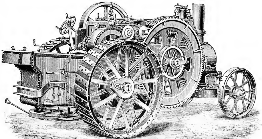
3. Dampfpluglokomotive mit senkrechter Seitrommel von Sack in Leipzig-Plagwitz.
