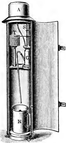
Fig. 6. Pluviograph von Hellmann-Zueß.
