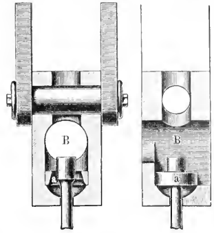
3a. Einlegevorrichtung.
