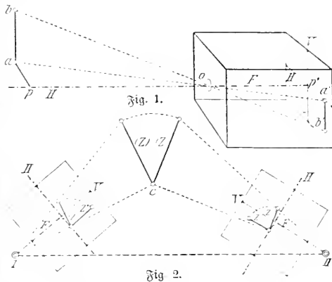
Fig. 1 u. 2. Meßbildverfahren.
