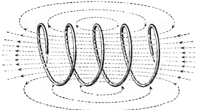
Fig. 2. Kraftlinien in einer vom Strom durchflossenen Drahtspule.
