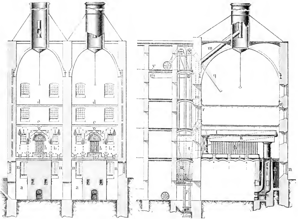
2. Malzdarre von Tanner u. Laetsch.
