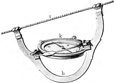
Marktscheiderkompaß.
