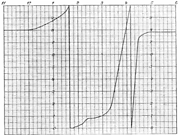
Fig. 7. Registrierprobe des Hellmannschen Pluviographen.
