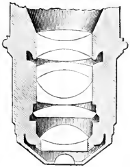
2c. Objektiv.
