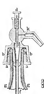
Fig. 1. Garnitur der Siphonflasche.
