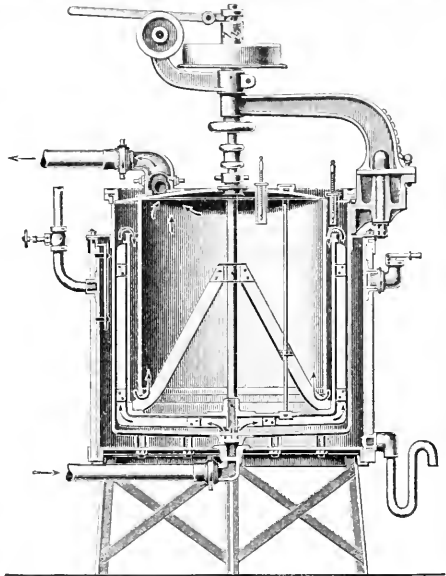
3. Regenerativmilcherhitzer von Lefeldt u. Lentsch.
