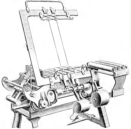
3. Abschneideapparat von Leinhaas.
