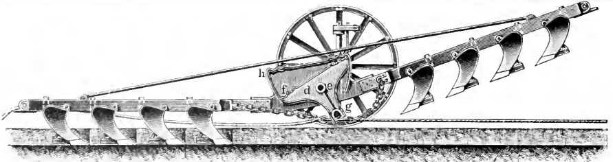
1. Kippflug von A. Ventzki in Graudenz.
