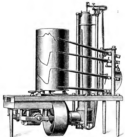
Fig. 12. Baro-Thermo-Hygrograph von Hergesell und Bosh.
