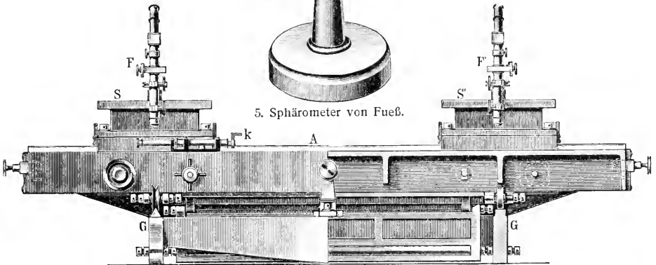
2. Komparator von Bamberg, hintere Ansicht.
