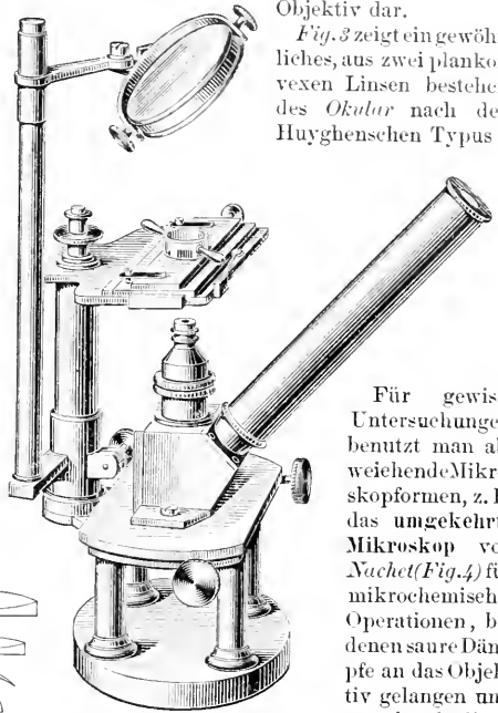
4. Umgekehrtes Mikroskop.
