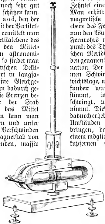
Fig. 2. Magnetometer (gleiches Spiegelgalvanometer).
