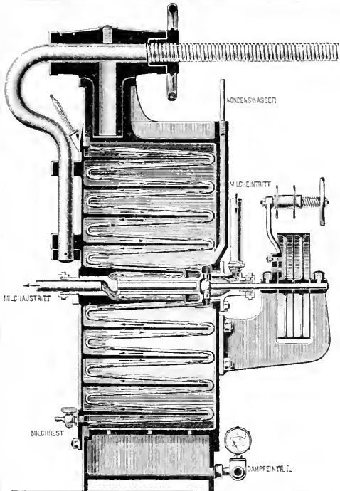
2. Bergedorfer Pasteurisierungsapparat.
