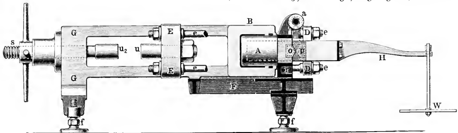
Fig. 2. Werder'sche Maschine.
