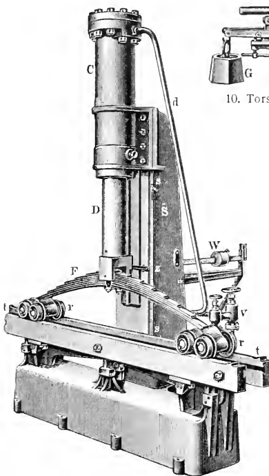
11. Hydraulische Federprüfungsmaschine.
