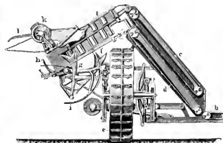
6. Bindemäher der Deering Harvester Comp., Chicago. Querschnitt
