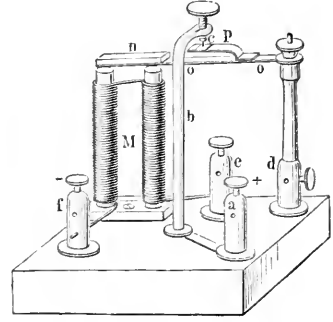
Wagner'scher Hammer
