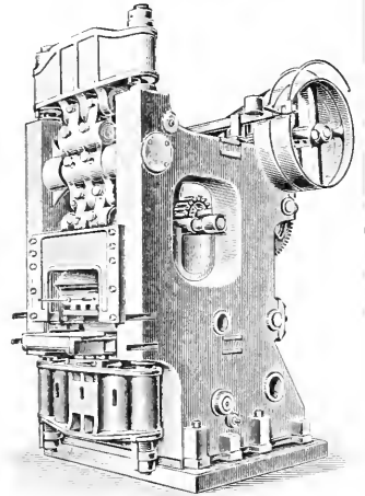
5. Trockenpresse der Aktiengesellschaft Tigler.
