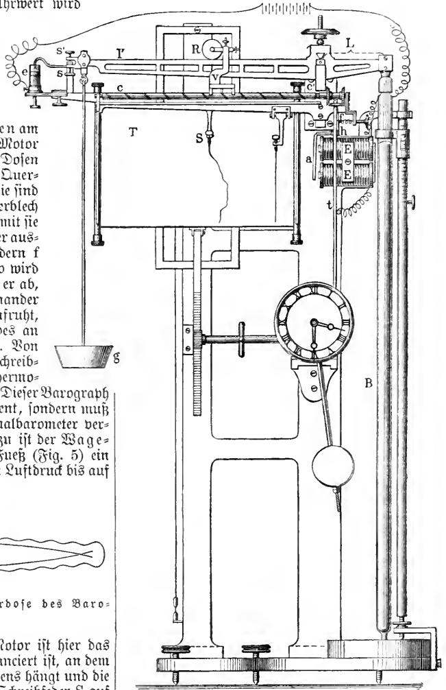
Fig. 5. Wagebarograph von Sprung- und Fuß.
