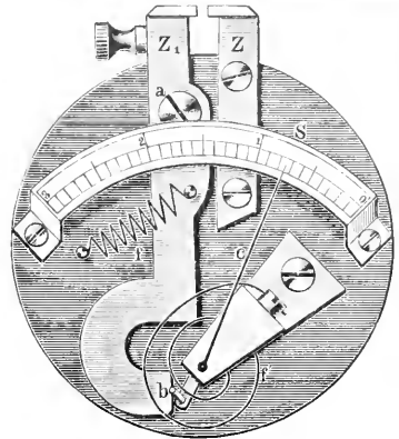
4. Mikrometertaster von Fueß.
