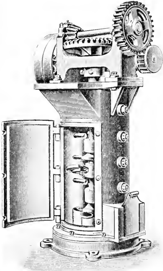
2. Tonschneider von Laeis u. Komp.
