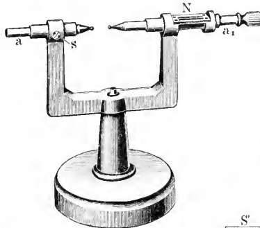
5. Sphärometer von Fueß.
