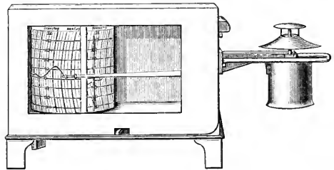
Fig. 1. Thermograph von Hfmann = Fuez.
