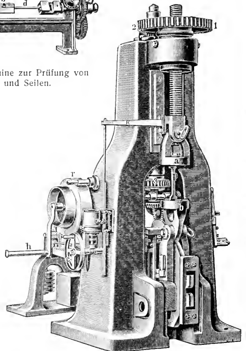
6. Zerreiβmaschine mit Schraubkraft.
