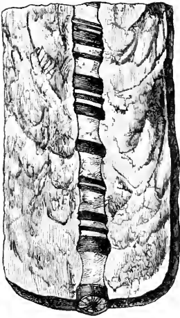
3. Gestreckter Belemnit.
