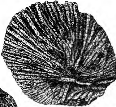
8. Querschnitt durch ein Chondrum, stark vergrößert.
