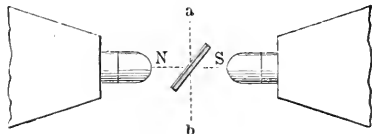
Fig. 4. Diamagnetismus.
