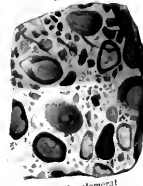
21 Konglomerat
