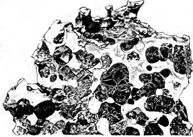
5. Pallas-Eisen.
