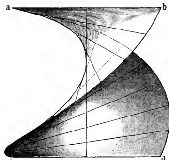
Fig. 1. Gemeine Schraubenfläche.
