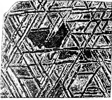
1. Toluca-Eisen.
