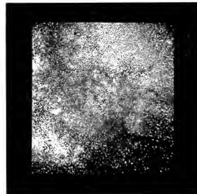
5. zwischen Trifid-Nebel und \theta Ophiuchi (R. A. 17h 10m, Dekl. -23^{\circ} , 26. Juni 1895);
