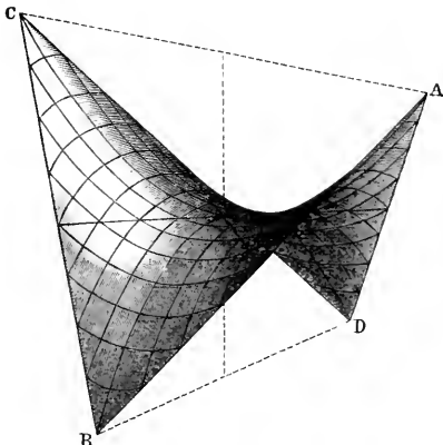
Fig. 2. Schwarz'sche Minimalfläche.
