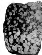
17 Struktur in glasigem Gestein
