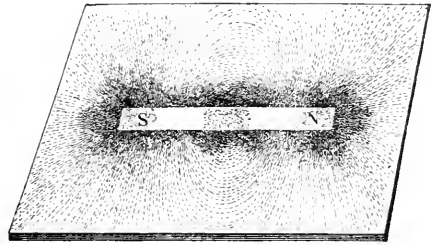
Fig. 2. Magnetische Kraftlinien.
