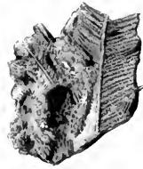
8 Gestrichelte Kristalle
