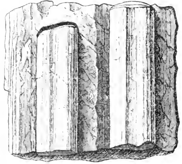
5. Stylolithen.
