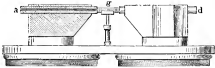
Diamagnetische Drehung der Polarisationsebene des Lichtes.
