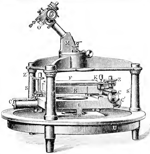
3. Apparat zur Ausmessung von Himmelsphotographien von Repsold.
