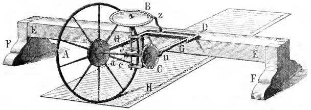
Fig. 1. Meßapparat.
