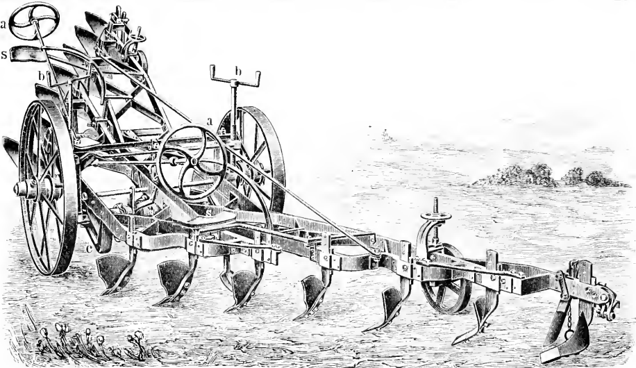
1. Siebenfurchenkipplpflug mit Antibalance-Vorrichtung von J. Fowler u. Comp. in Leeds.
