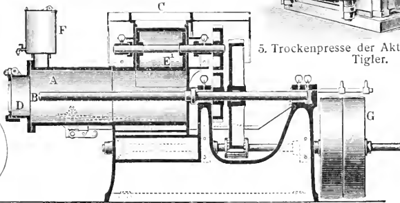
6. Schlickeysens liegende Ziegelpresse. Quer- und Längsschnitt.
