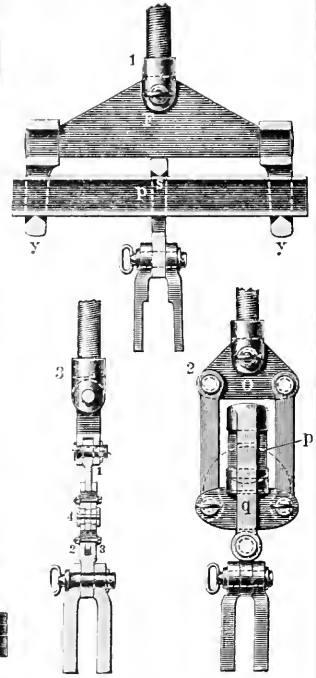
8. Einspannvorrichtungen (1, 2 u. 3).
