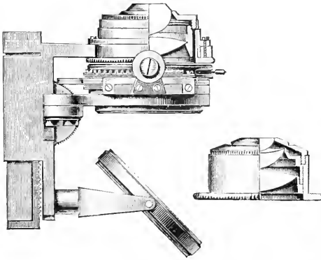
18. Abbesscher Apparat.
