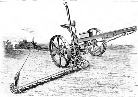
2. Grassmähdmaschine der Erzgebirgischen Maschinenfabrik in Schleitzau.
