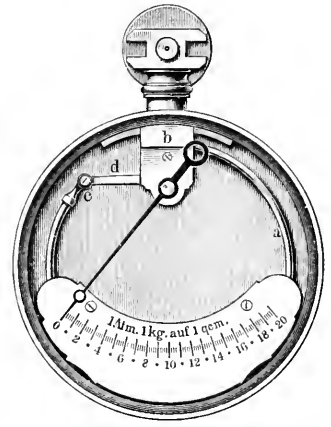
Fig. 3. Röhrenfedermanometer.
