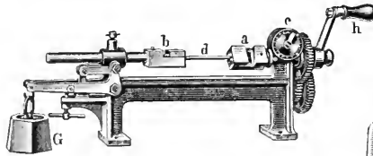
10. Torsionsmaschine zur Prüfung von Drähten und Seilen.
