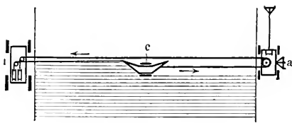
Fig. 3. Einmaschinenystem.
