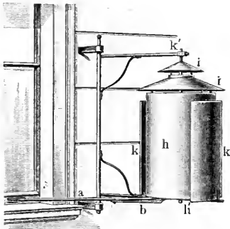
Fig. 2. Preussisches Thermometergehäuse.
