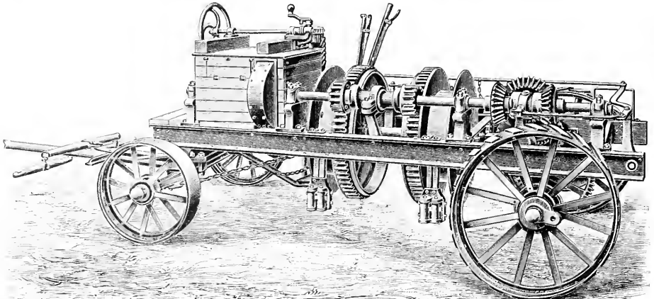
4. Motorwagen für das elektrische Einmaschinensystem von Eckert in Berlin.
