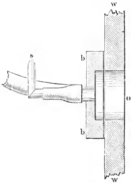
Fig. 4. Manometrische Kapsel.
