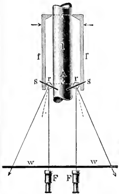
1. Spiegelapparat zum Messen der Formänderungen.
