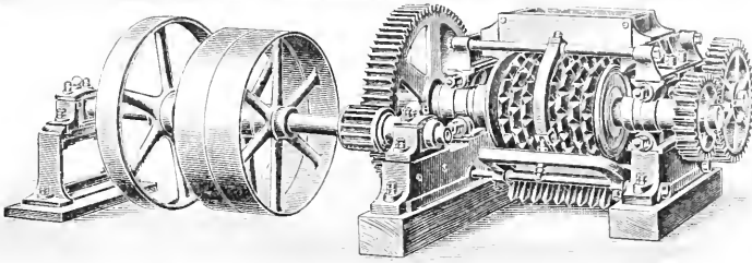
1. Riffelbrechwalze von Schlickeysen.
