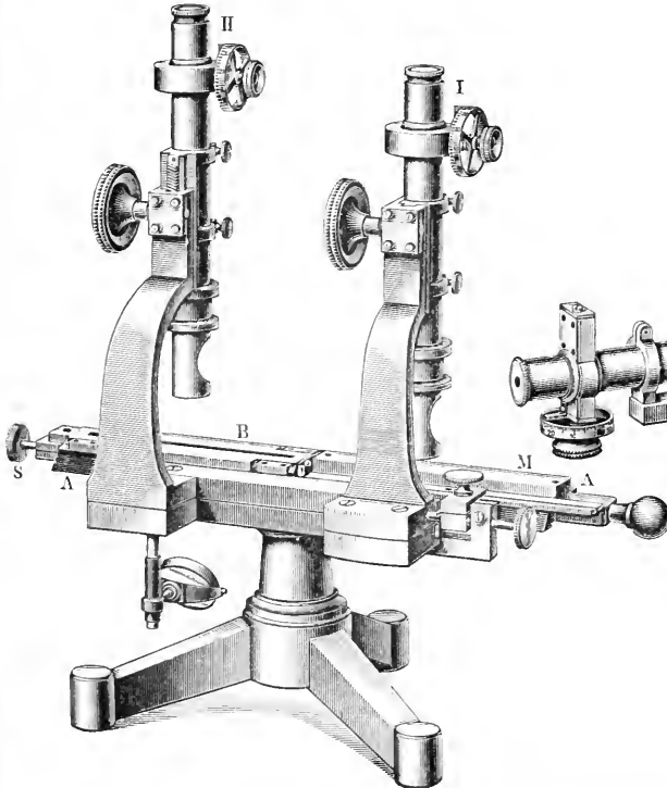
4. Komparator von Zeiß.
