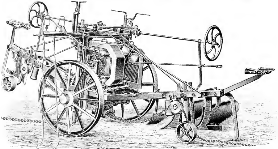
3. Elektrischer Pflug von F. Zimmermann u. Komp. in Halle a. S.
