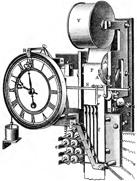
Fig. 8. Schreibapparat des Anemographen von Sprung-Zueß.
