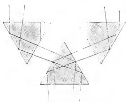
8. Trennung der Strahlenbündel im Binokular-Mikroskop.
