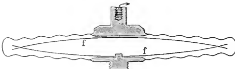
Fig. 4. Querschnitt einer Federdose des Barographen.
