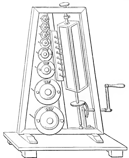
Fig. 6. Resonatoren-Flammenapparat.
