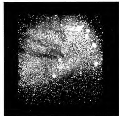
6. bei Antares (R. A. 16h 20m, Dekl. -23^{\circ} , 30. März 1895).
