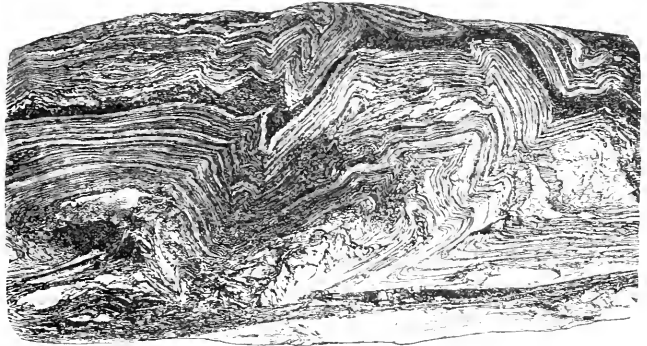
6. Gefältelter Schiefer.
