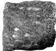
18 Mandelsteinstruktur
