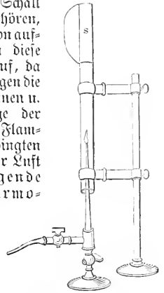
Fig. 1. Singende Flamme.
