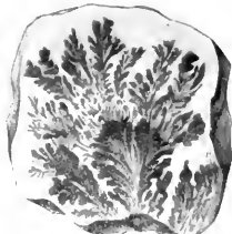
6 Dendritische Mineralbildung
