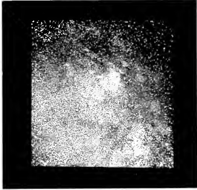
1. Region bei Messier II (R. A. 18h 40m, Dekl. -8^{\circ} , 16. August 1895);
