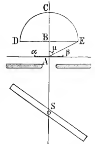
Fig. 2. Darstellung der numerischen Apertur.
