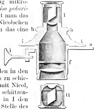
15. Polarisations-vorrichtung.
