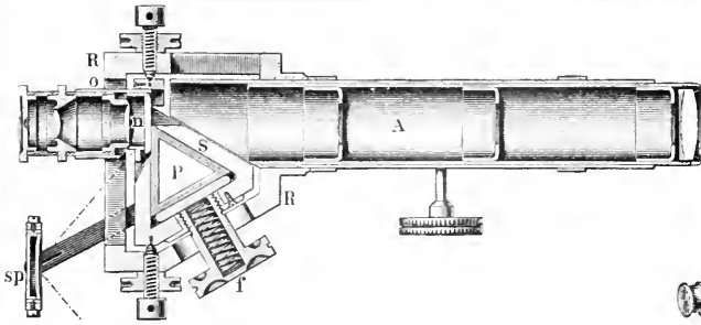
1. Horizontalschnitt durch das Fernrohr von Fig. 2.
