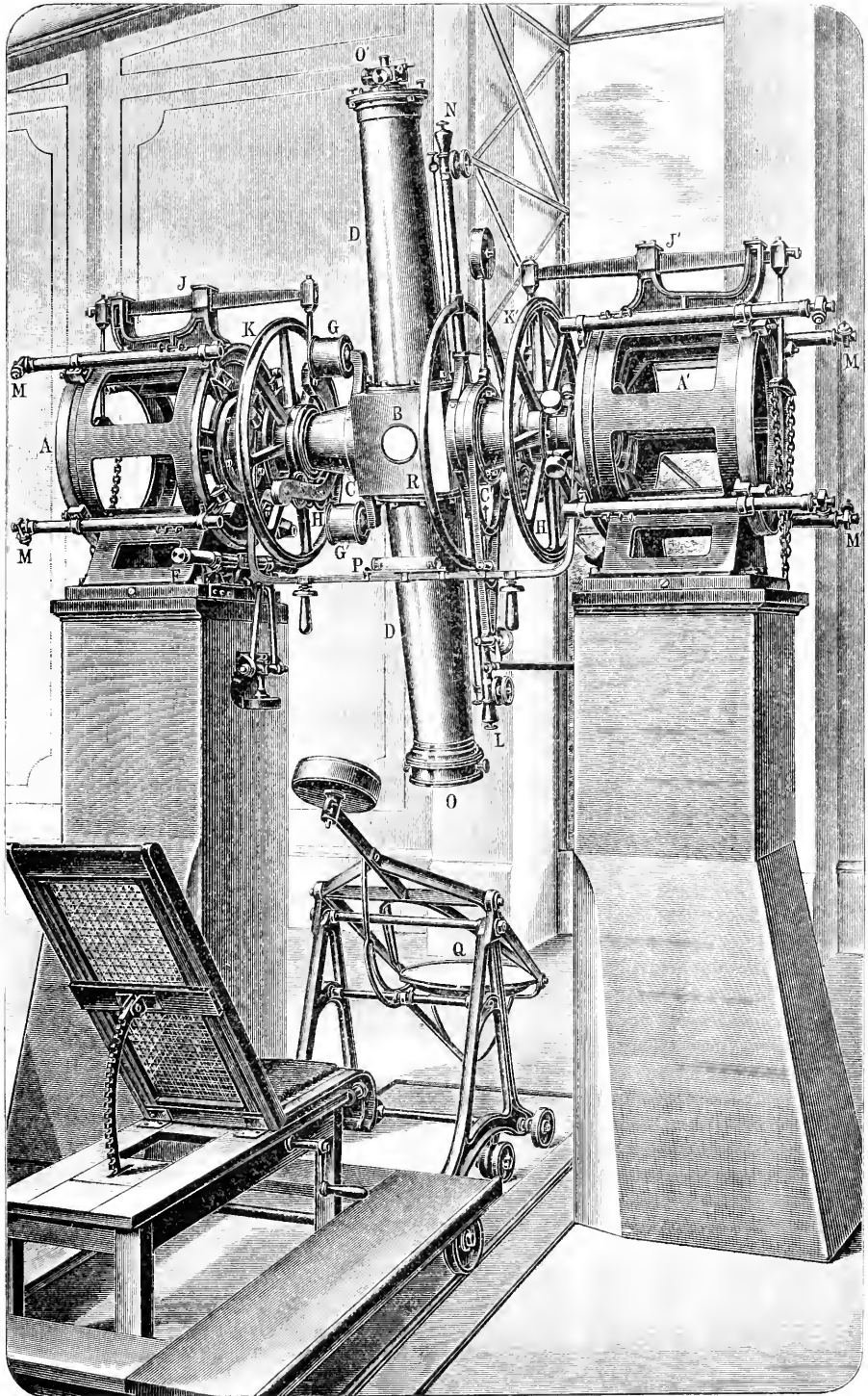
Meridiankreis der Sternwarte in Straßburg.
