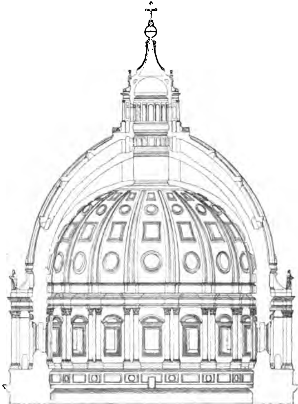
Abb. 98. Durchschnitt von Michelangelos Modell für die Kuppel der St. Peterkirche in Rom. (Zu Seite 110.)
