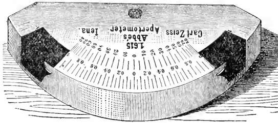
FIG. 165. Abbe Apertometer.
