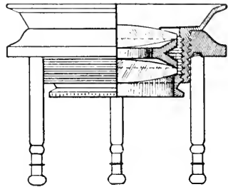
FIG. 201. TRIPOD MAGNIFIER.
