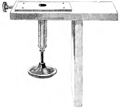
FIG. 389.—Simple microtome.
