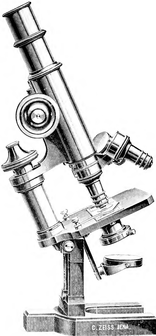
FIG. 190.—Zeiss's stand VLA (1898).
