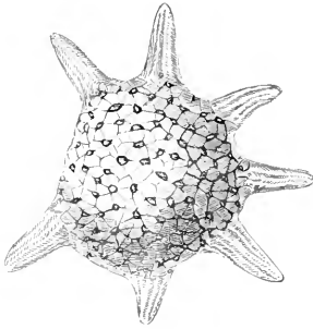
FIG. 623.— Tinoporus baculatus .
