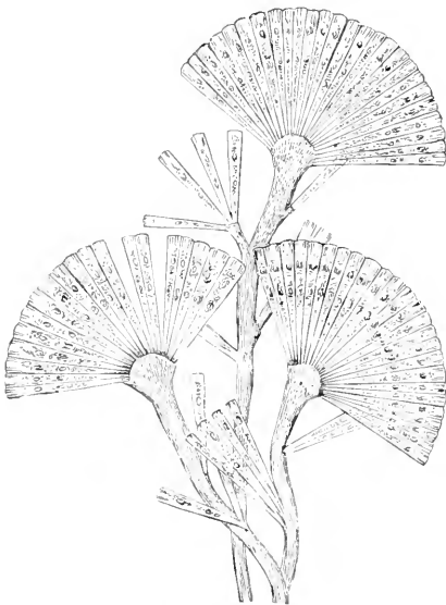
FIG. 450.— Licmophora flabellata .
