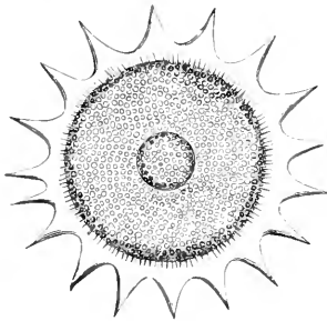
FIG. 651.— Haliomma Humboldtii .
