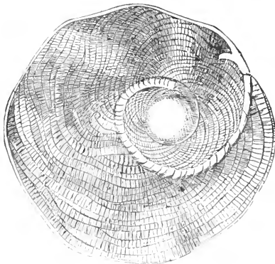
FIG. 635.— Heterostegina .
