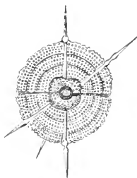
FIG. 650.— Stylodyctya gracilis .
