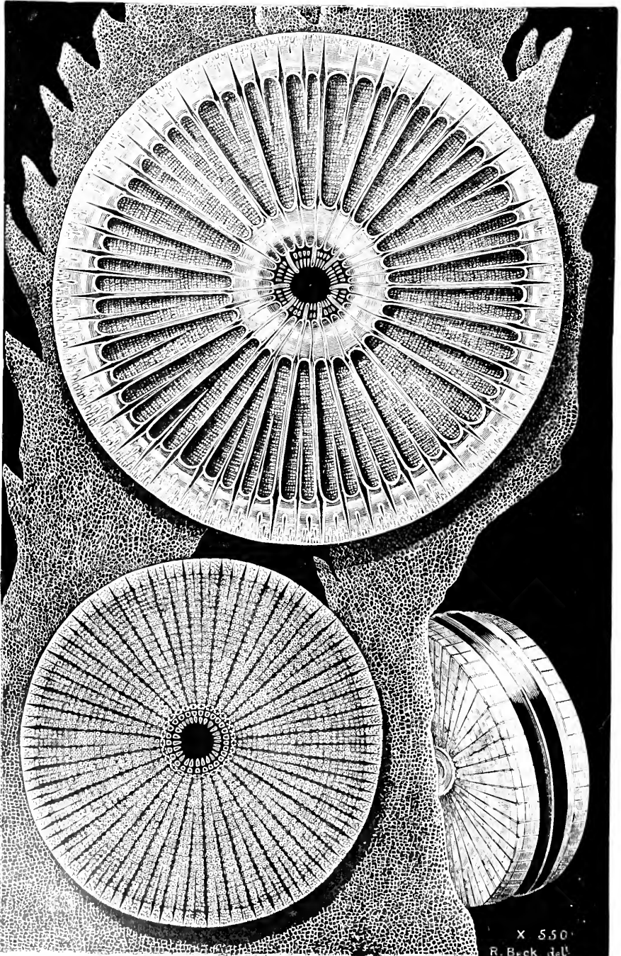
ALCHINOSITES JAPONICUS.
