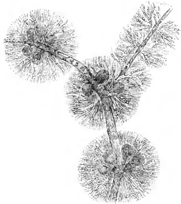
FIG. 433. Batrachospermum moniliforme .
