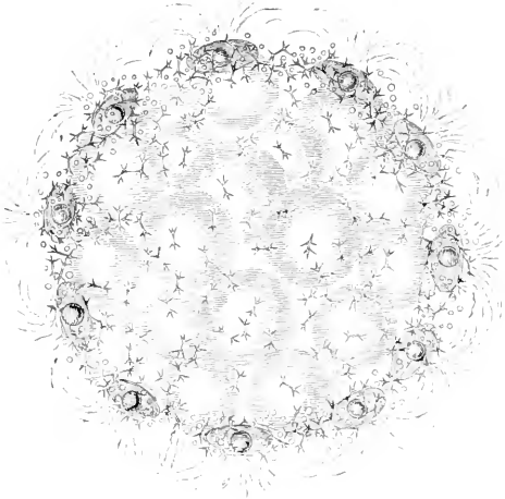
FIG. 652.— Spharozoum ovoidimare .
