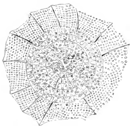
FIG. 649.— Perichlamyditium praeertum .
