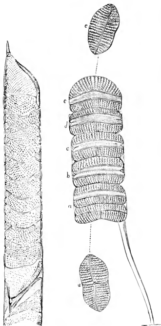
FIG. 460.— Rhizosolenia imbricata .
