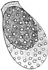
FIG. 603. Ehippial egg.
