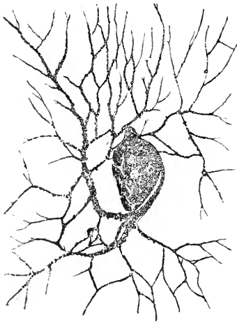
FIG. 570.— Lieberkuehnia Wageneri .
