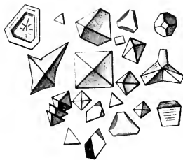
Fig. 22. Kaliumchloroplatinat-Kristalle. Vergr. 285.
