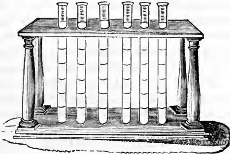
Fig. 72. Lactometer.
