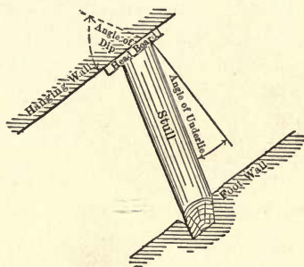
FIG. 44. — STULL.
