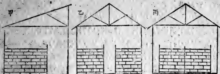
圖 16 荔枝干焙爐建築形式示意圖
