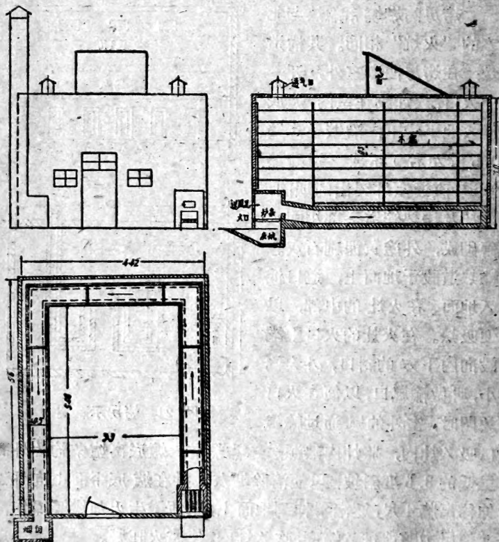
圖 22 北京果脯廠烤房示意圖
