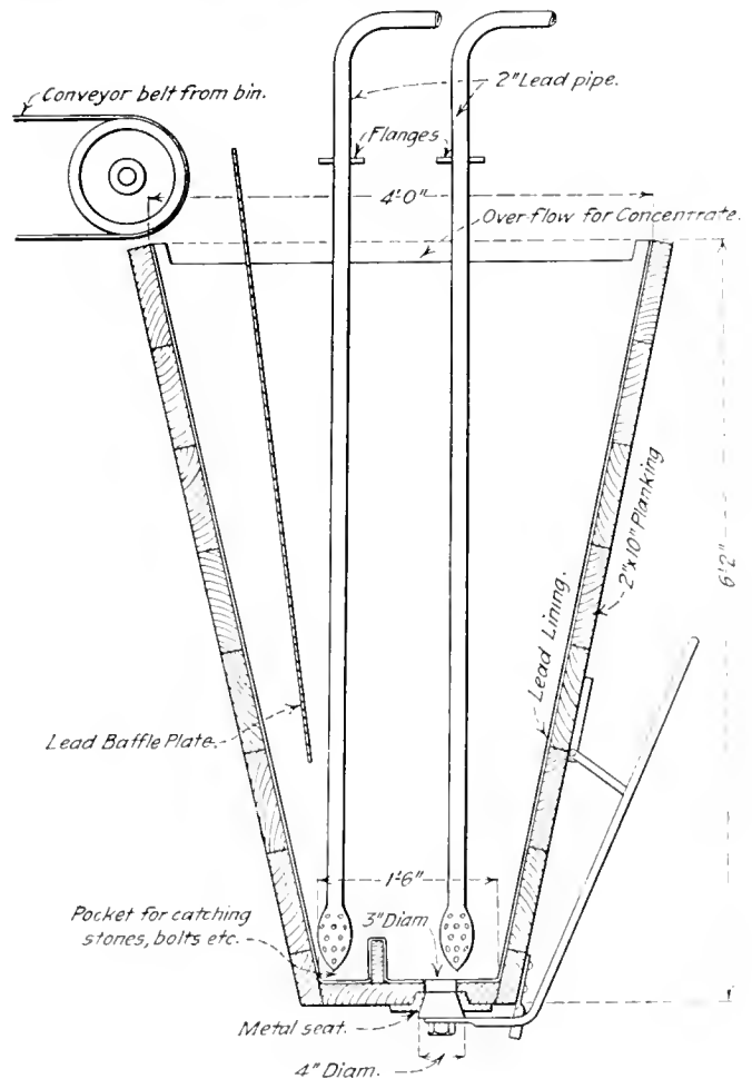
FIG. 10. THE POTTER APPARATUS.
