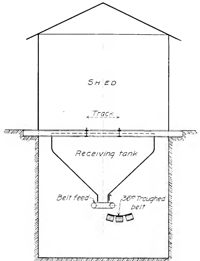
FIG. 9. UNLOADING BIN.
