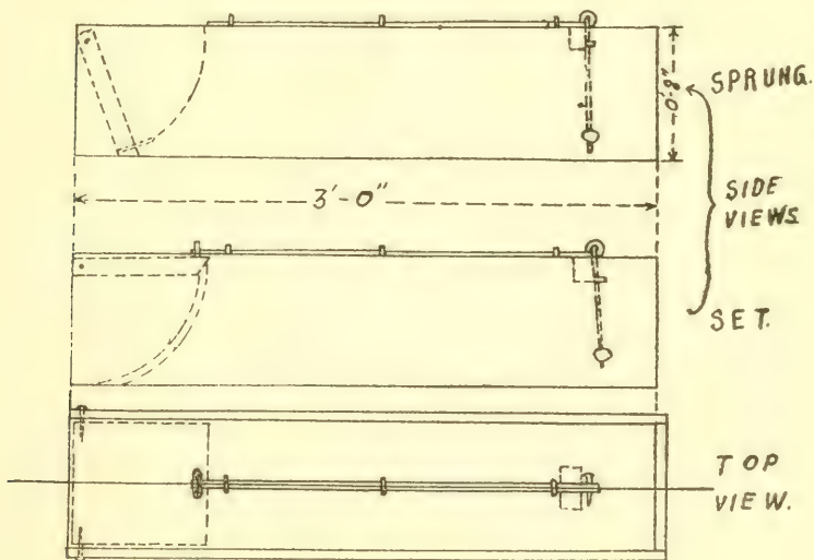
Fig. 2. BOX TRAP.
