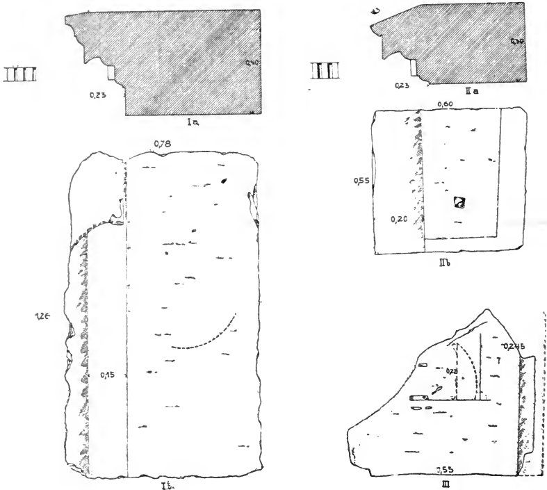
Fig. 5. — Altarpodium, Gesimsblöcke.
