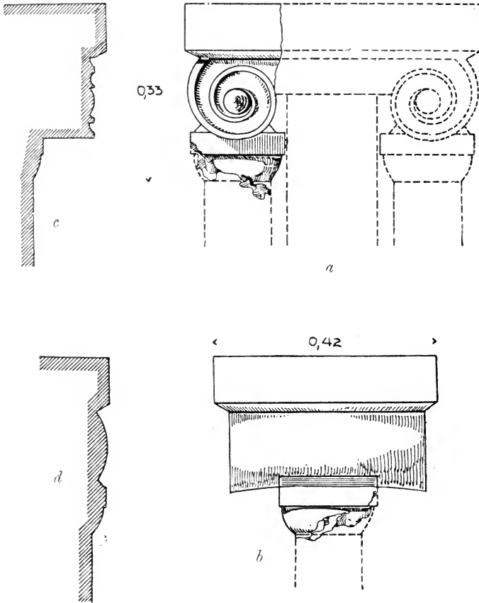
Fig. 17. — Opfertisch (Ergänztes punktiert). a. Front. b. Seite. c. Schnitt durch die Volute. d. Schnitt durch das Polster.
