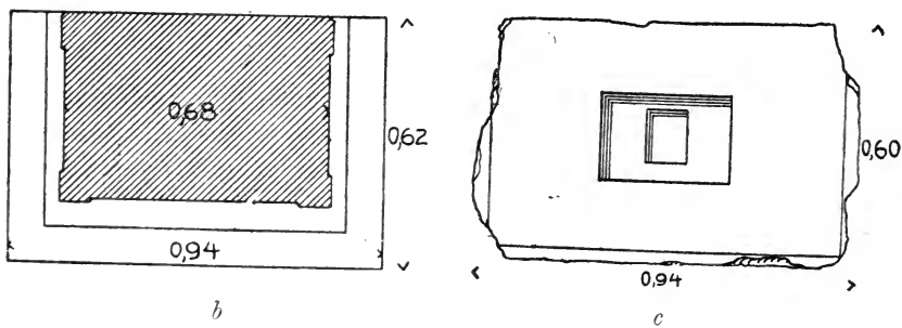
Fig. 21. — Ionischer Altar. a. Ansicht; links o. Profil in Stein, rechts o. Seite des Pilasterkapitells. b. Querschnitt. c. Aufsicht.
