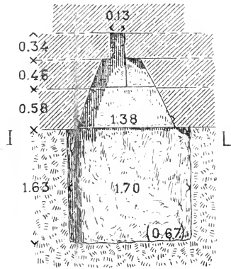
SEZIONE I-L
