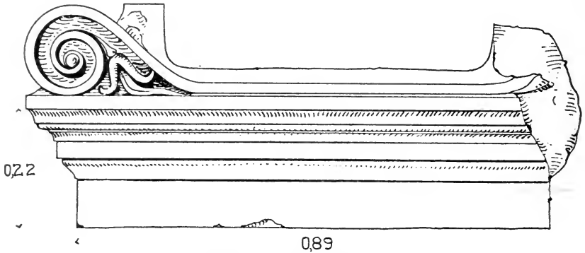
Fig. 20. — Altaraufsatz.
