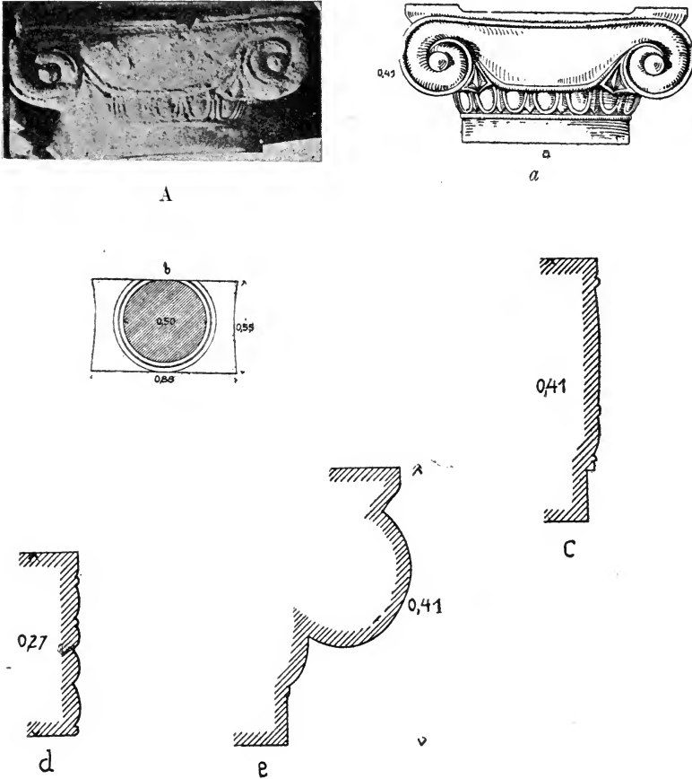
FIG. 12. — Ionisches Kapitell.
