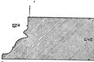
Fig. 3. — Altarpodium, Sockelprofil.
