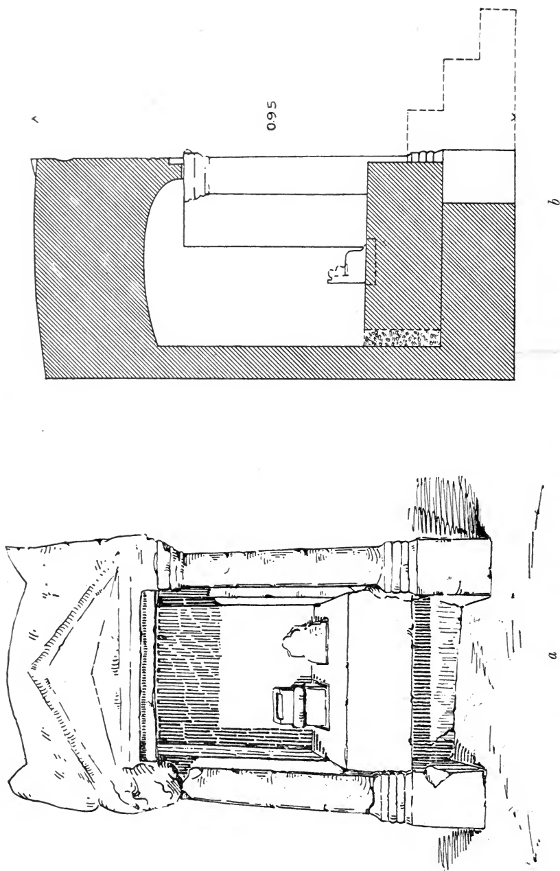
Fig. 11. — Aedicula. a. Ansicht. b. Schnitt durch die Mitte. (Ergänztes punktiert).
