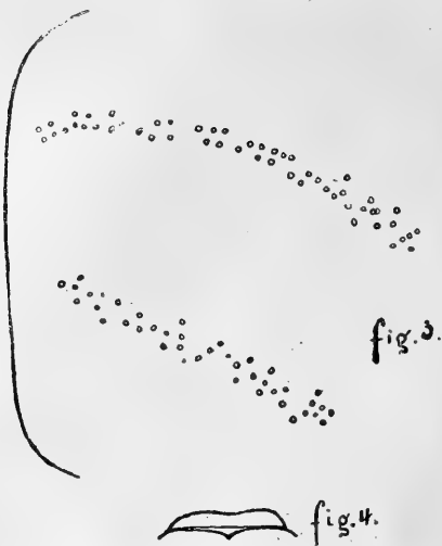
Fig. 3. — Séries antéro-externe et médio-externe chez Neosternolophus artensis MONTR. Fig. 4. — Echancrure du clypeus chez le même.
