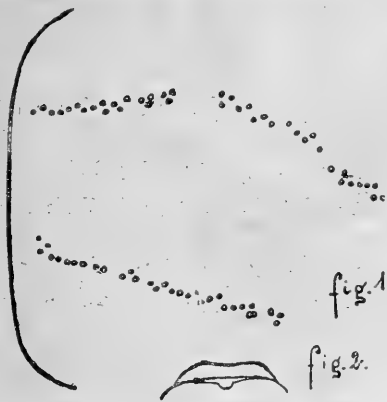
Fig. 1. — Séries antéro-externe et médio-externe chez Neost. tenebricosus BLACKB.
