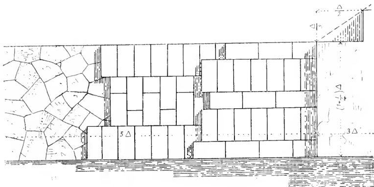
Fig. 19 bis. — Detail des murs de liaison.
