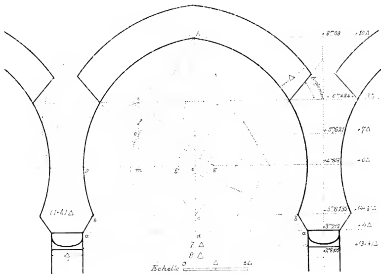
Fig. 11. — Épure de la voûture.
