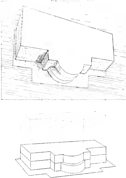
Fig. 4. — Première assise de la pile-culée n° 3, XV. Au fond de la fouille. Ramenée au niveau du sol.
