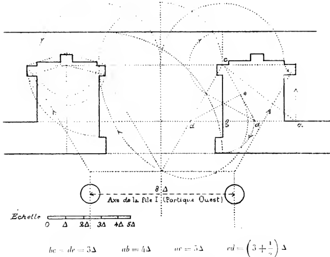
Fig. 16. — Épure du plan des porches.
