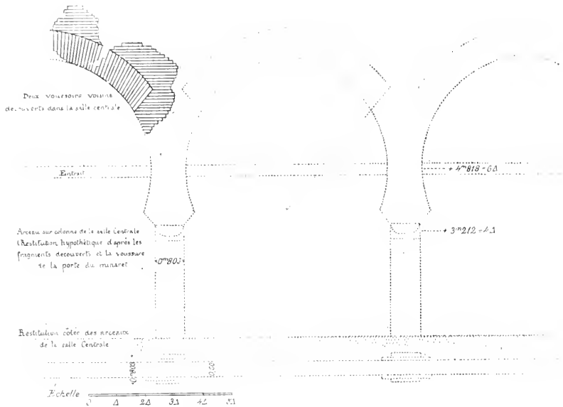
Fig. 70. — Restitution cotée des arceaux de la salle Centrale.
