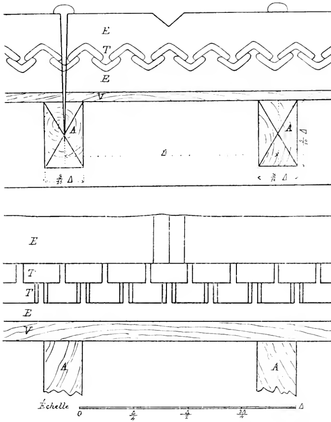
Fig. 75. — Coupe longitudinale de la toiture par un plan normal à la ligne de plus grande pente et projection horizontale de la toiture décomposée en ses diverses conches.
