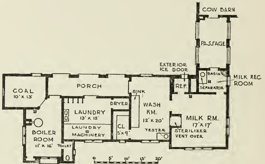
FIG. 23—DAIRY AT OAKDALE, L. I., FOR F. G. BOURNE, ESQ.
