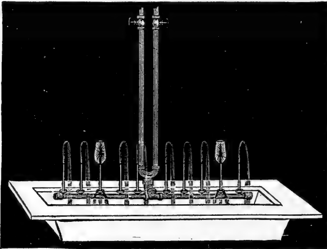
FIG. 23—TEST-BOTTLE RINSER
