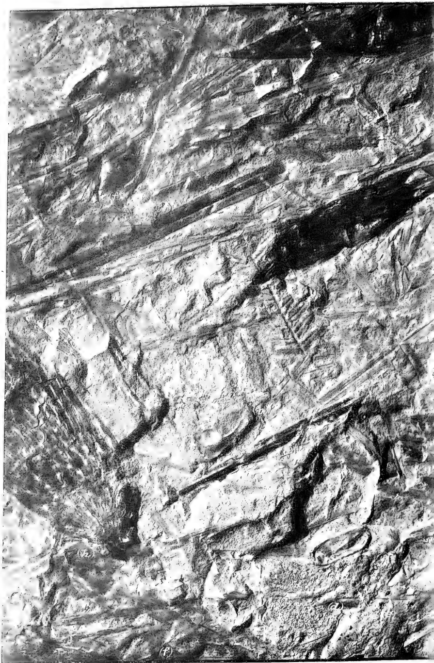
FERNS: CALLIPTERIDIUM. LYCOPODIALES: LEPIDOSTROBUS, LEPIDOPHYLLUM, LE
