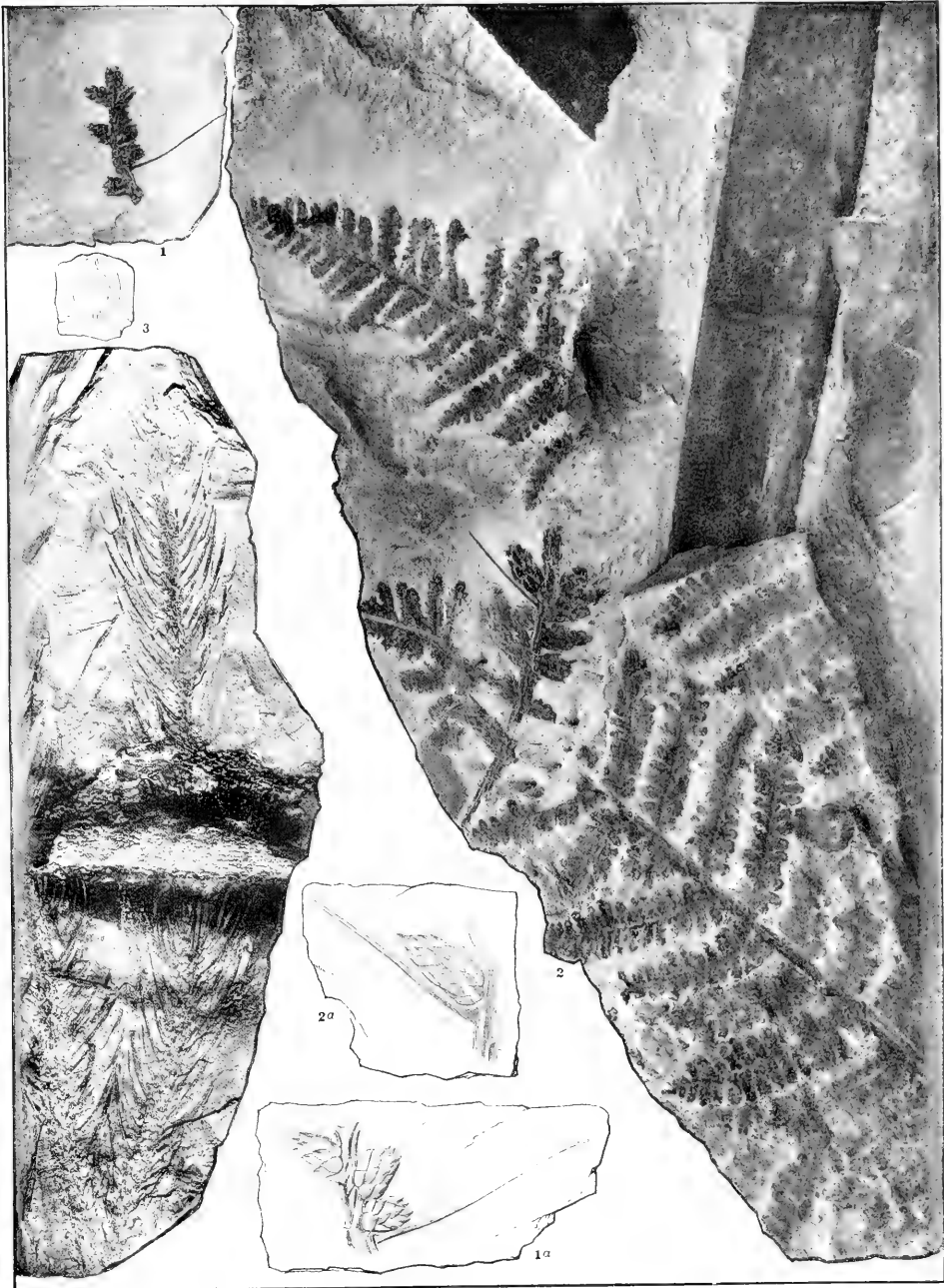
FERNS: PECOPTERIS. LYCOPODIALES: LEPIDODENDRON. CORDAITALES: CORDAITES, CORDAIANTHUS, AND CARDIOPARON.
