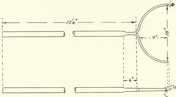
Fig. 69. RING-SHIFTER
