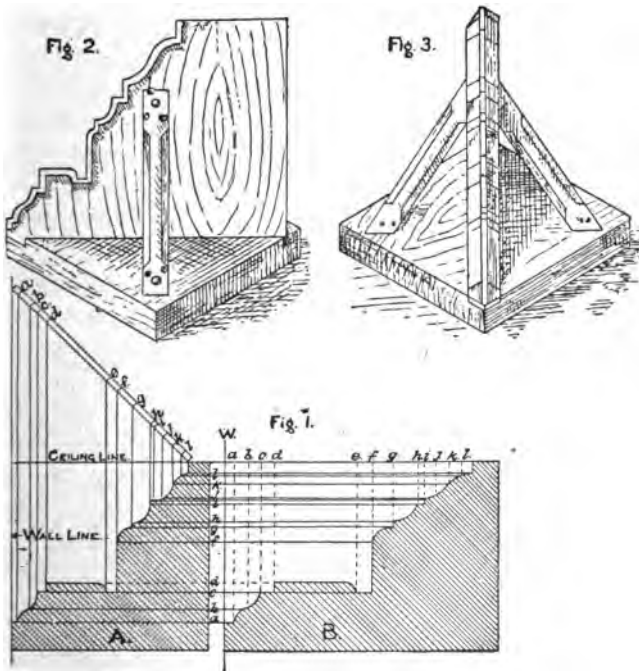
-MITRE-MOULD.
