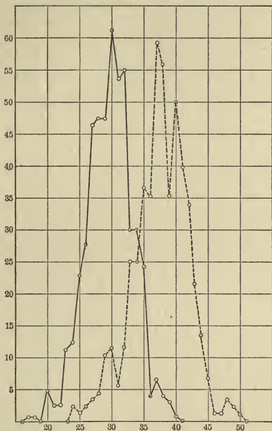
FIG. 7. Variation in leaf-width of Onagra rubrinervis and O. lamarekiana . O. rubrinervis : R., 17 to 40 mm.; M., 29.736 \pm 0.098 mm.; \sigma , 3.559 \pm 0.069 mm.; C. V., 12.07 \pm 0.23 per cent. O. lamarekiana : R., 24 to 50 mm.; M., 37.617 \pm 0.137 mm.; \sigma , 4.248 \pm 0.097 mm.; C. V., 11.29 \pm 0.26 per cent.
