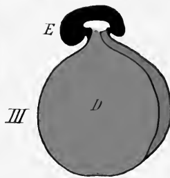
Allantoisplacentation
