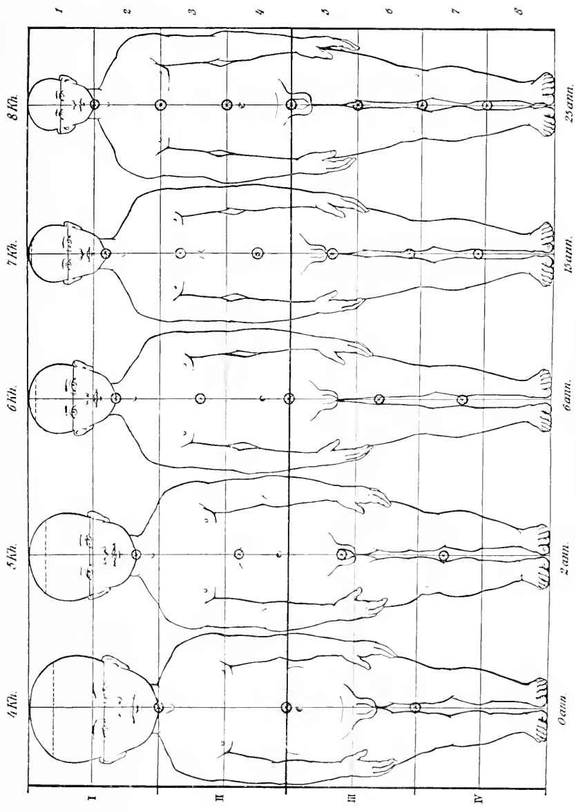
Fig. 82. Wachstumsproportionen.
