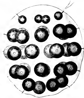
PLEODORINA
