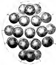
EUDORINA
