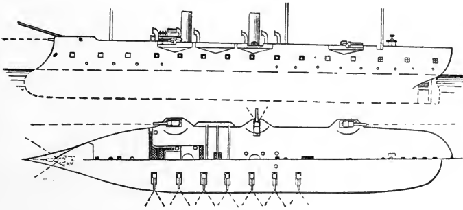
TOURVILLE.
