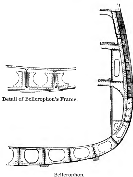
Bellerophon.
