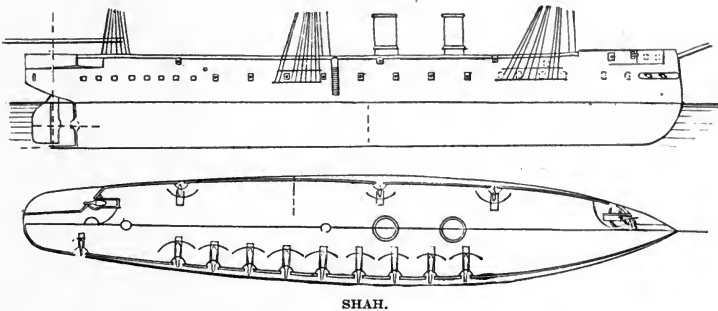
SHAH.
