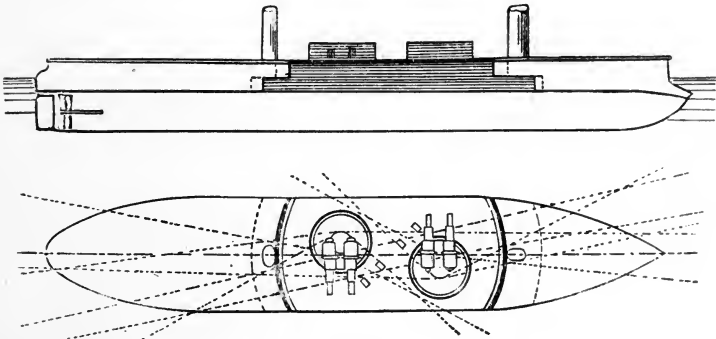
DUILIO.
