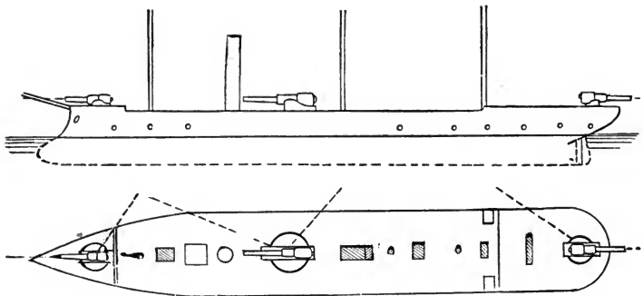
LYNX.
