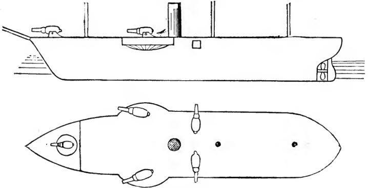
JORGE JUAN.
