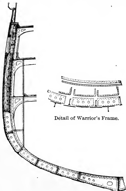
Warrior.
