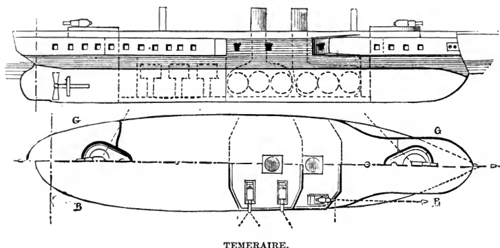
TEMERAIRE.
