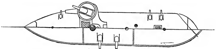
VICTORIEUSE.
