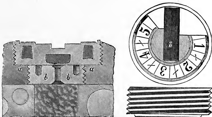
Bormann Fuse.
