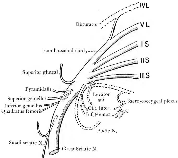
FIG. 304.—Sacral plexus.
