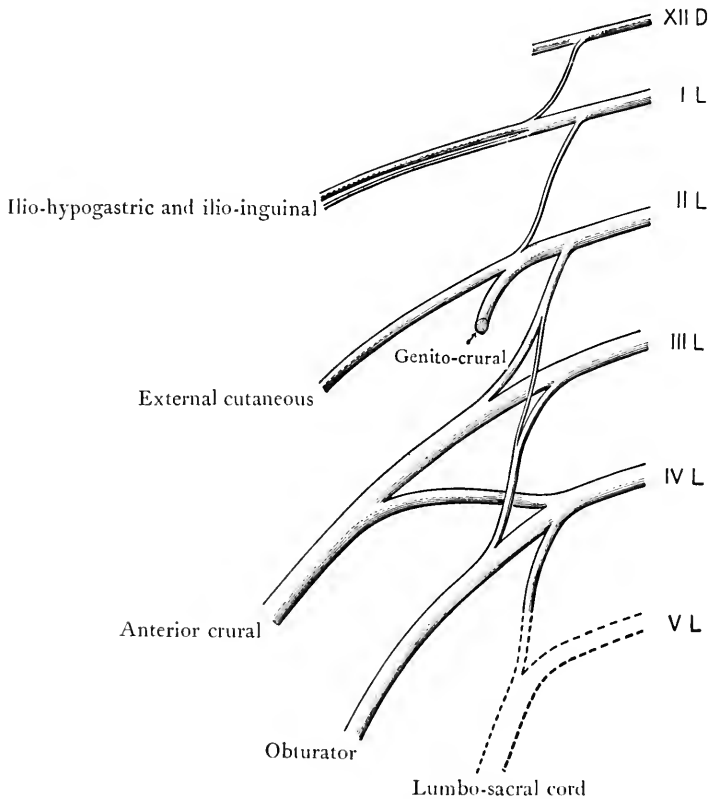
FIG. 301.—Lumbar plexus.
