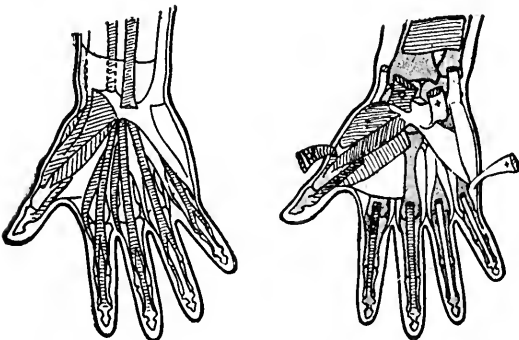
FIG. 149.—Superficial layer.
