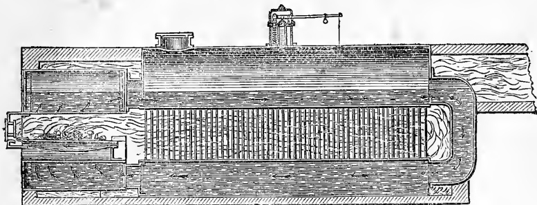
LONGITUDINAL SECTION.
