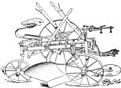
FIG. 5. SULKY PLOW.
