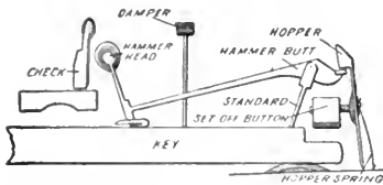
STREICHER'S GRAND PIANOFORTE ACTION.
