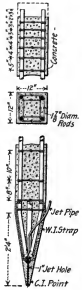
CONCRETE-STEEL PILE.
