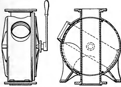
SENDING APPARATUS. -
