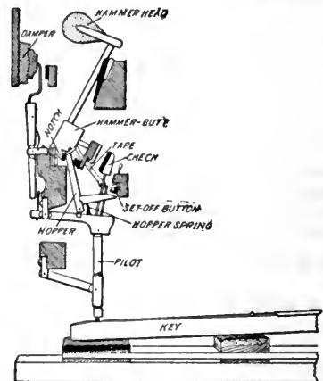
ENGLISH UPRIGHT PIANOFORTE ACTION.
