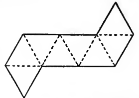
OCTAHEDRON.
