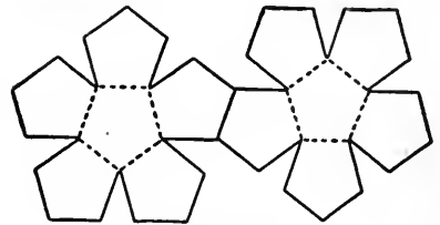
DODECAHEDRON.
