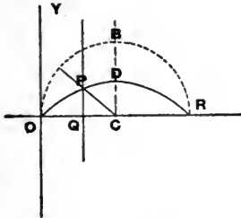
QUADRATRIX.
