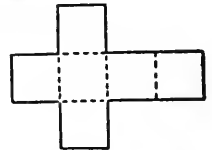
HEXAHEDRON.
