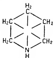
Piperidine.
