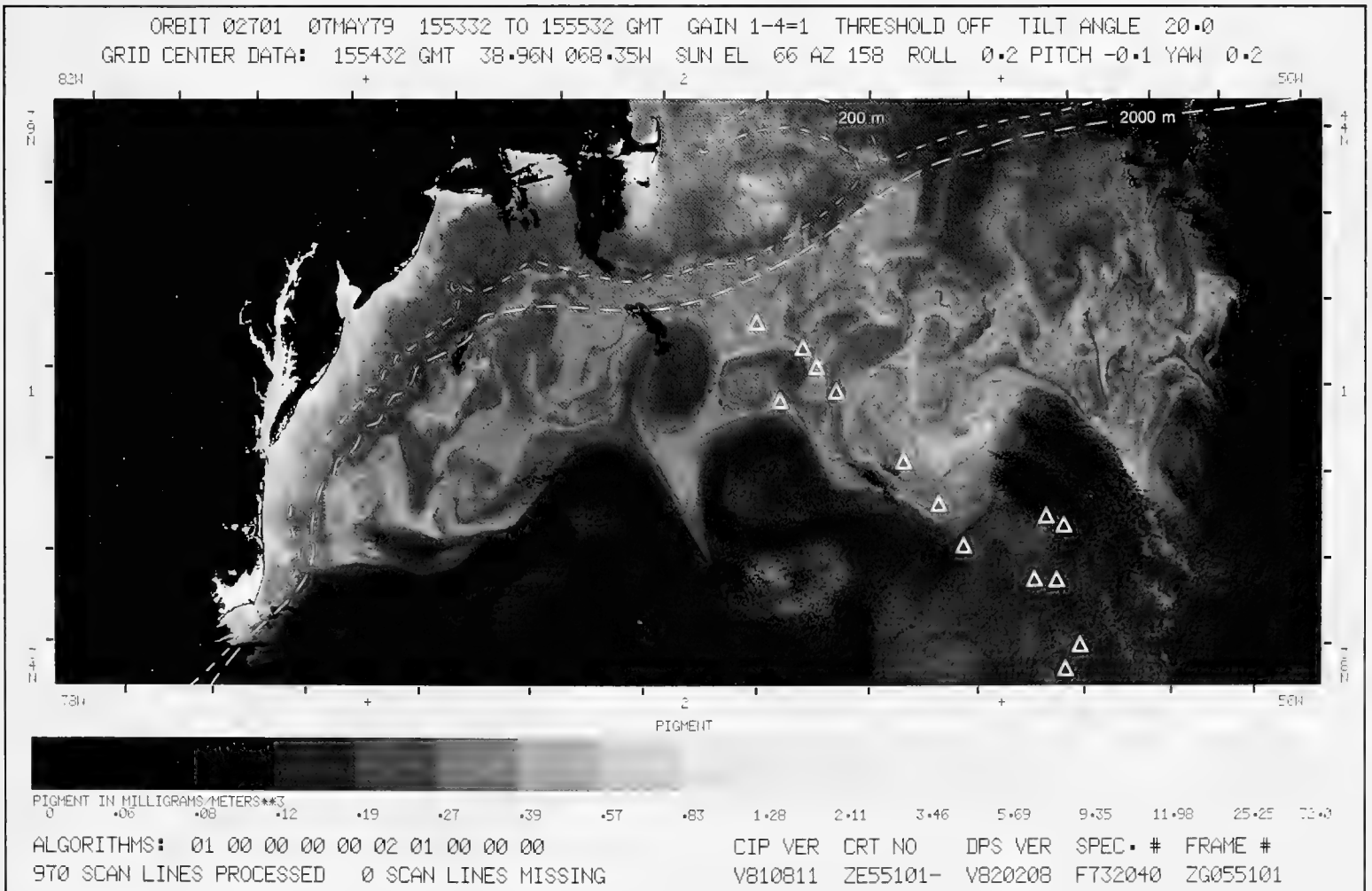
55-2. Nimbus-7. Orbit 2701. 7 May 1979. CZCS Pigment Image.
