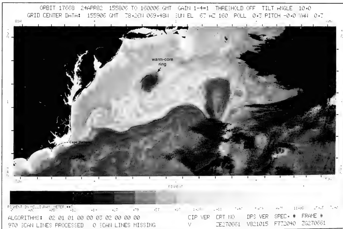
42-2. Nimbus-7. Orbit 17668. 24 April 1982. CZCS Pigment Image.
