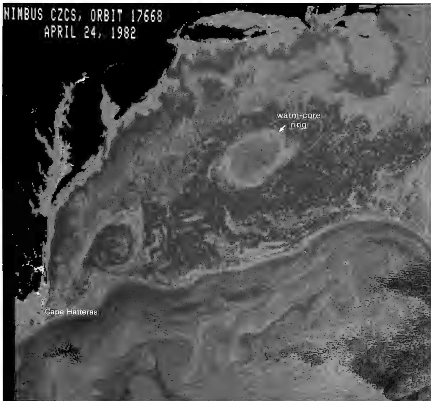
43-1. Nimbus-7. Orbit 17668. 24 April 1982. CZCS False-Color Pigment Image.
