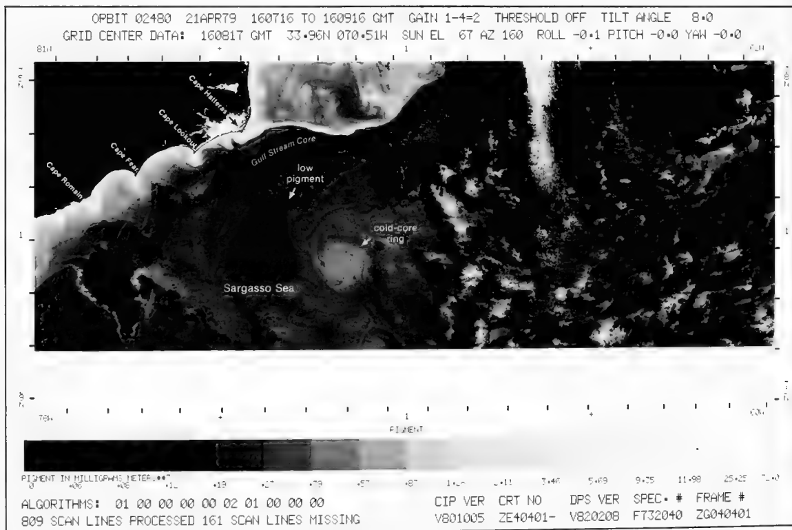
36-1. Nimbus-7. Orbit 2480. 21 April 1979. CZCS Pigment Image.
