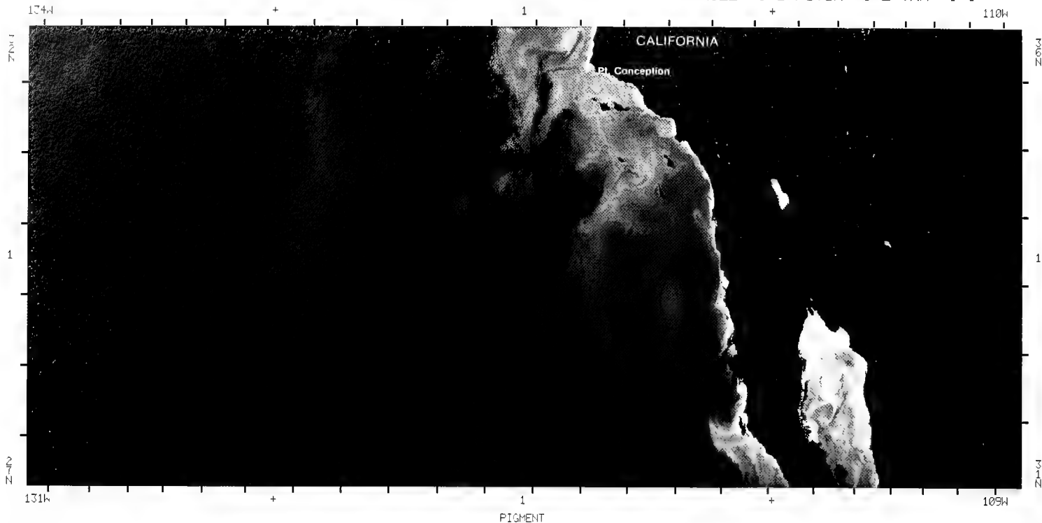
16-1. Nimbus-7. Orbit 2247. 4 April 1979. CZCS Pigment Image.
