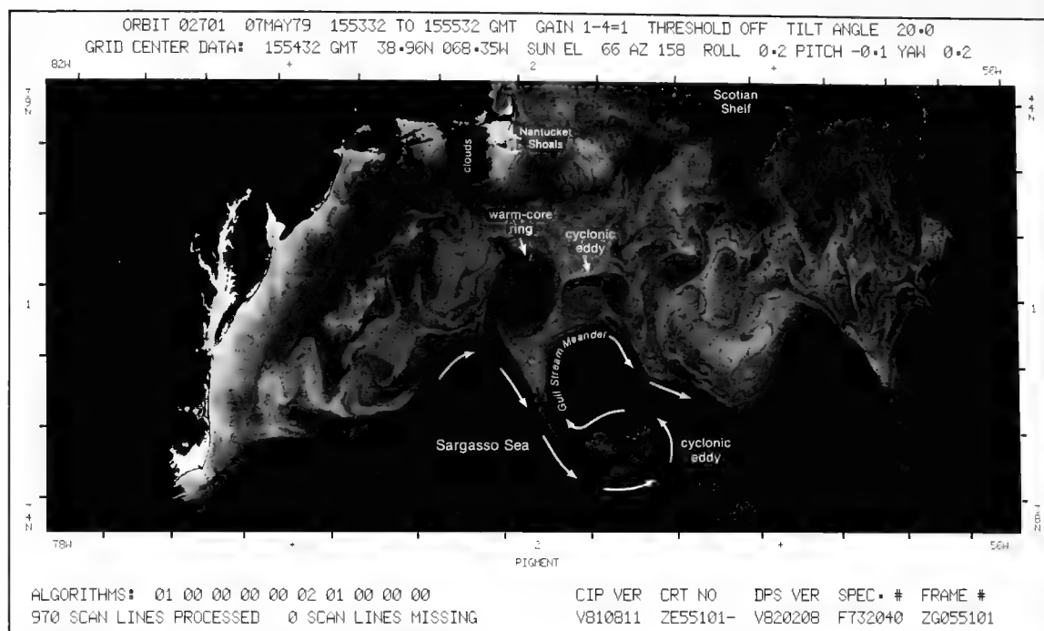
38-1. Nimbus-7. Orbit 2701. 7 May 1979. CZCS Pigment Image.
